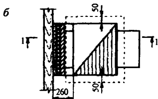
Рис. 2.3. Устройство закрытой отступки:
