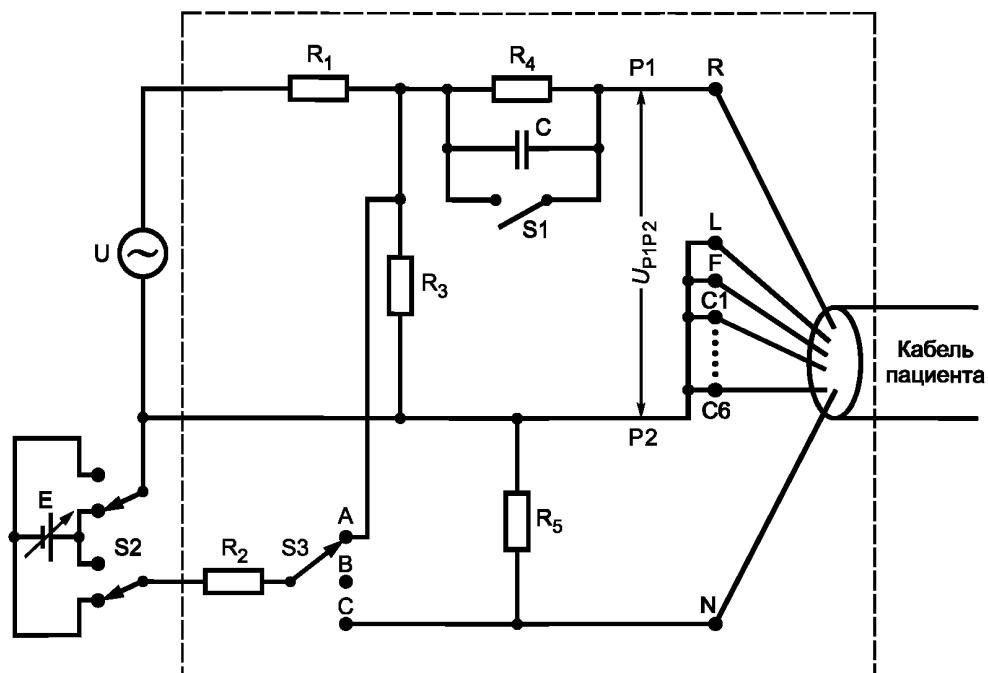
Генератор U должен иметь изолированный выход. При испытании ЭЛЕКТРОКАРДИОГРАФОВ с РАБОЧЕЙ ЧАСТЬЮ ТИПА BF или CF экранирующий кожух может заземляться.
