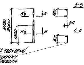
Схема стойки Г-Д1 (поз.1)
