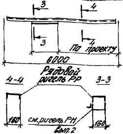
Схема ригеля РР-Д4 (поз.2)
