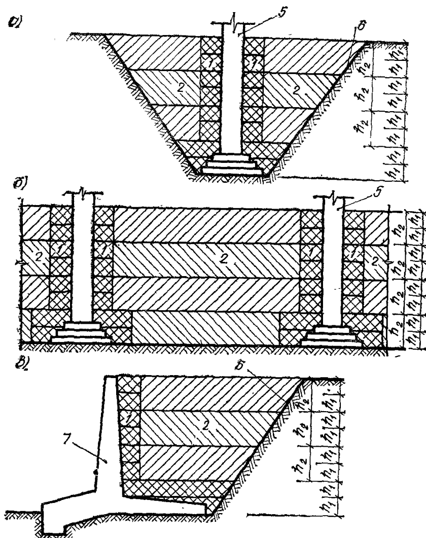
Рис. 1. Виды стесненных мест для обратных засыпок грунта
