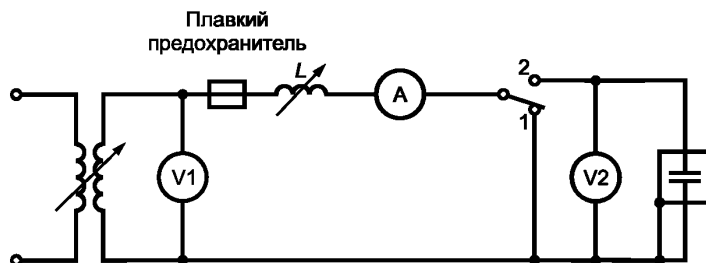
Рисунок 2 — Испытательная установка для разрушающего испытания переменным напряжением
