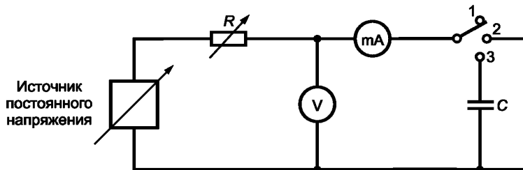
Рисунок 1 — Испытательная установка для выдержки при постоянном напряжении
