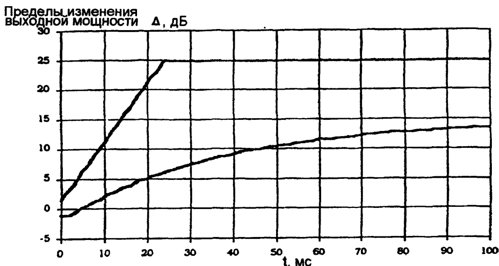
Рис.4.2.4.2.1. Шаблон изменения выходной мощности при \Delta P_{\text{в}}=20 дБ
