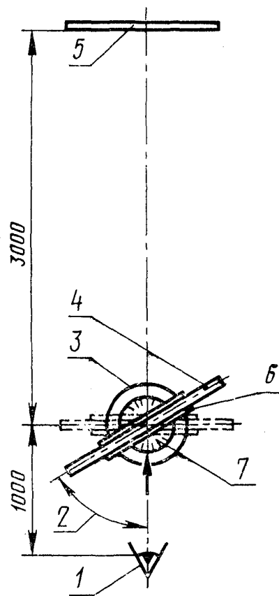
1—наблюдатель; 2—угол просмотра; 3—поворотный стол; 4—образец; 5—экран «кирпичная стена»; 6—каретка; 7—лимба
