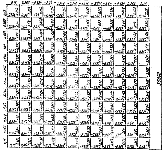
Схема усилий в нижних поясах и капиталах
