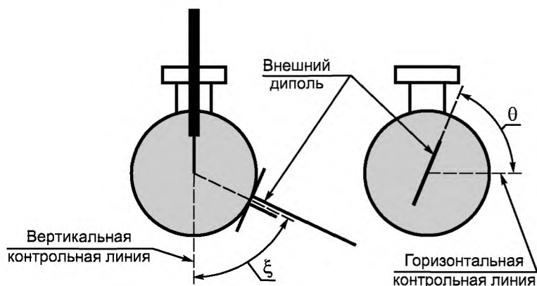
Рисунок В.6 — Условное обозначение положения \xi и поляризации диполя \theta [11]
