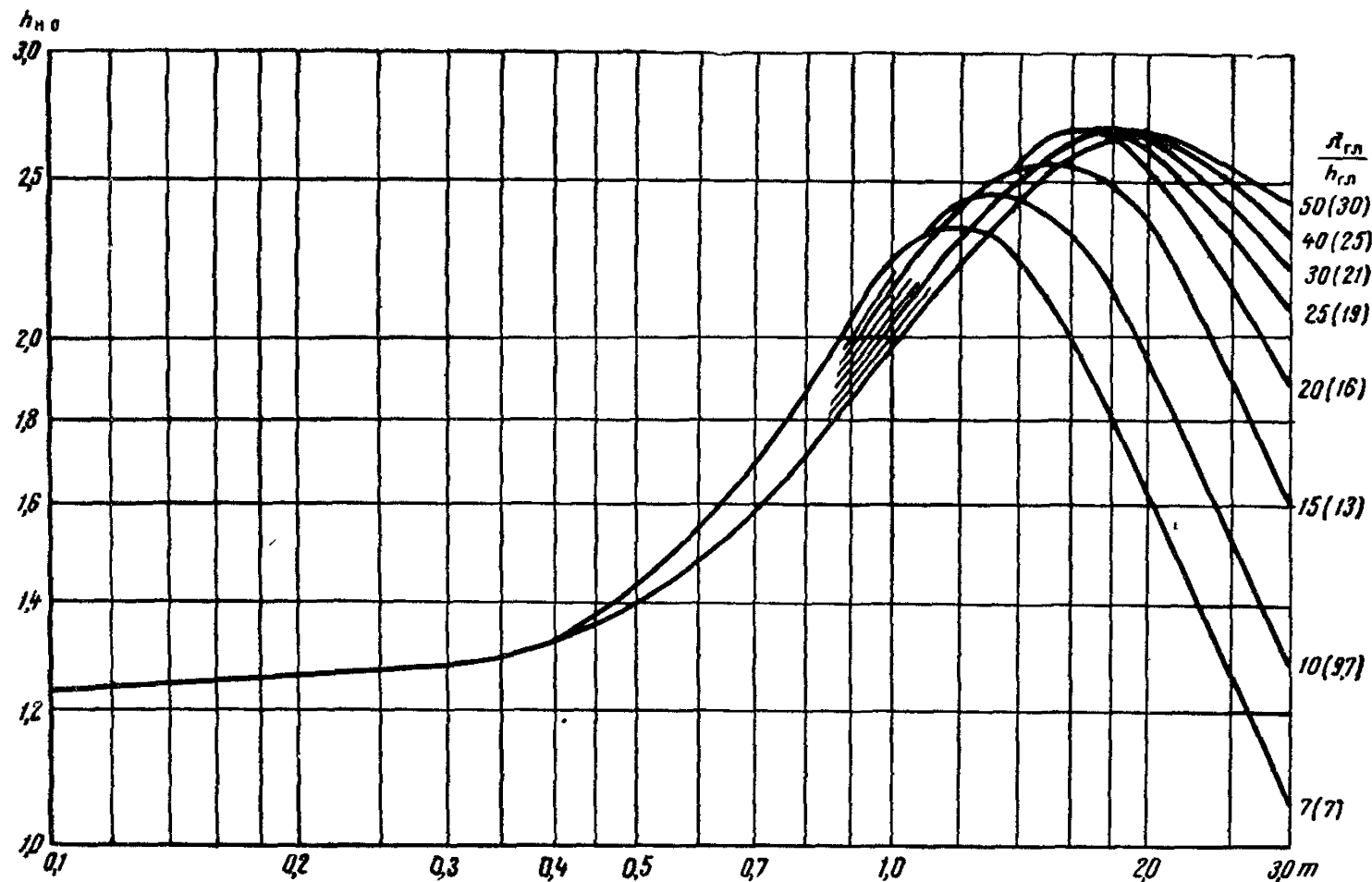
Рис. 19, а. Расчетная высота наката волн h_{нo} = h_{н1\%} в отношении к местной высоте волн при заложении откоса m \leq 3 (Значения шкалы пологостей волн, приведенные в скобках, принимаются при расчете наката по пологости волн на глубинах H = 2h )
