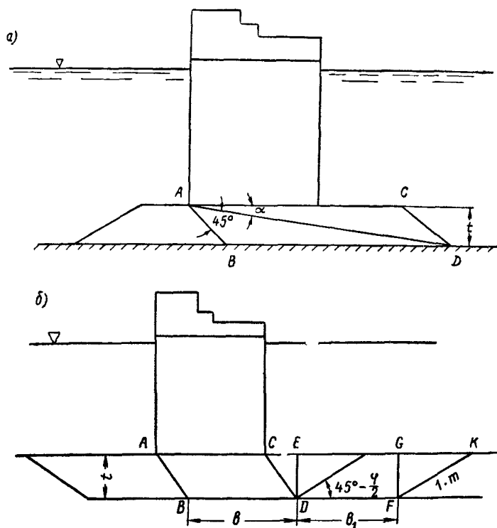
Рис 3 Схема расчета устойчивости сооружения на сдвиг a — постель находится на поверхности грунта основания, б — постель заглублена в грунт основания
