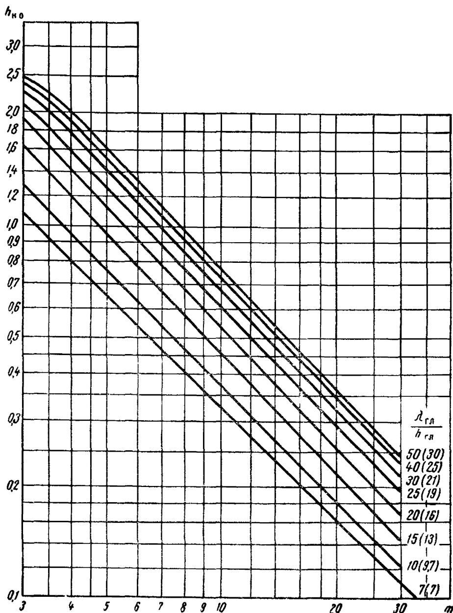
Рис. 19, б Расчетная высота наката волн h_{нo} = h_{н1\%} в отношении к местной высоте волн при заложении откоса m \geq 3 (Значения шкалы пологостей волн, приведенные в скобках, принимаются при расчете наката по пологости волн на глубинах H = 2h )
