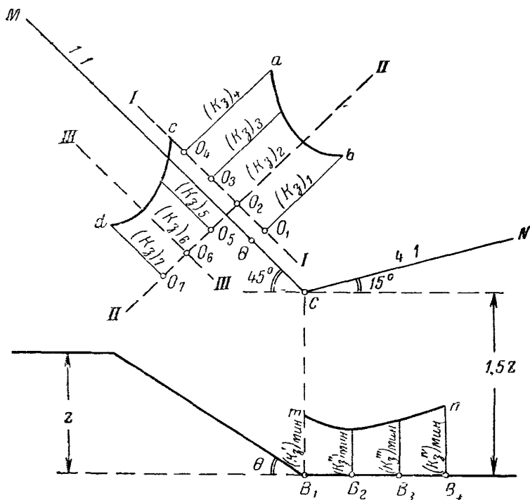
вертикали, проходящей через подошву откоса. Эта точка, как видно из рис. 45, возвышается над подошвой откоса на величину 1,5Z , где Z — высота откоса. Из найденной точки C проводим два луча, луч CM под углом 45^\circ к горизонту (в сторону откоса) и луч CN под углом 15^\circ (в противоположную сторону).
