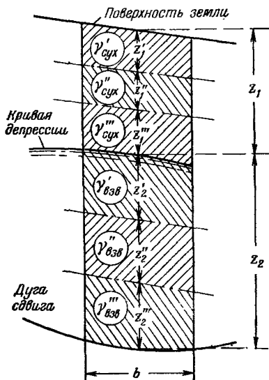
Решение. Пренебрегая весом пленочной воды в грунте, расположенном выше кривой депрессии, считаем, что объемный вес взвешенного грунта (см. формулу 1) равен
