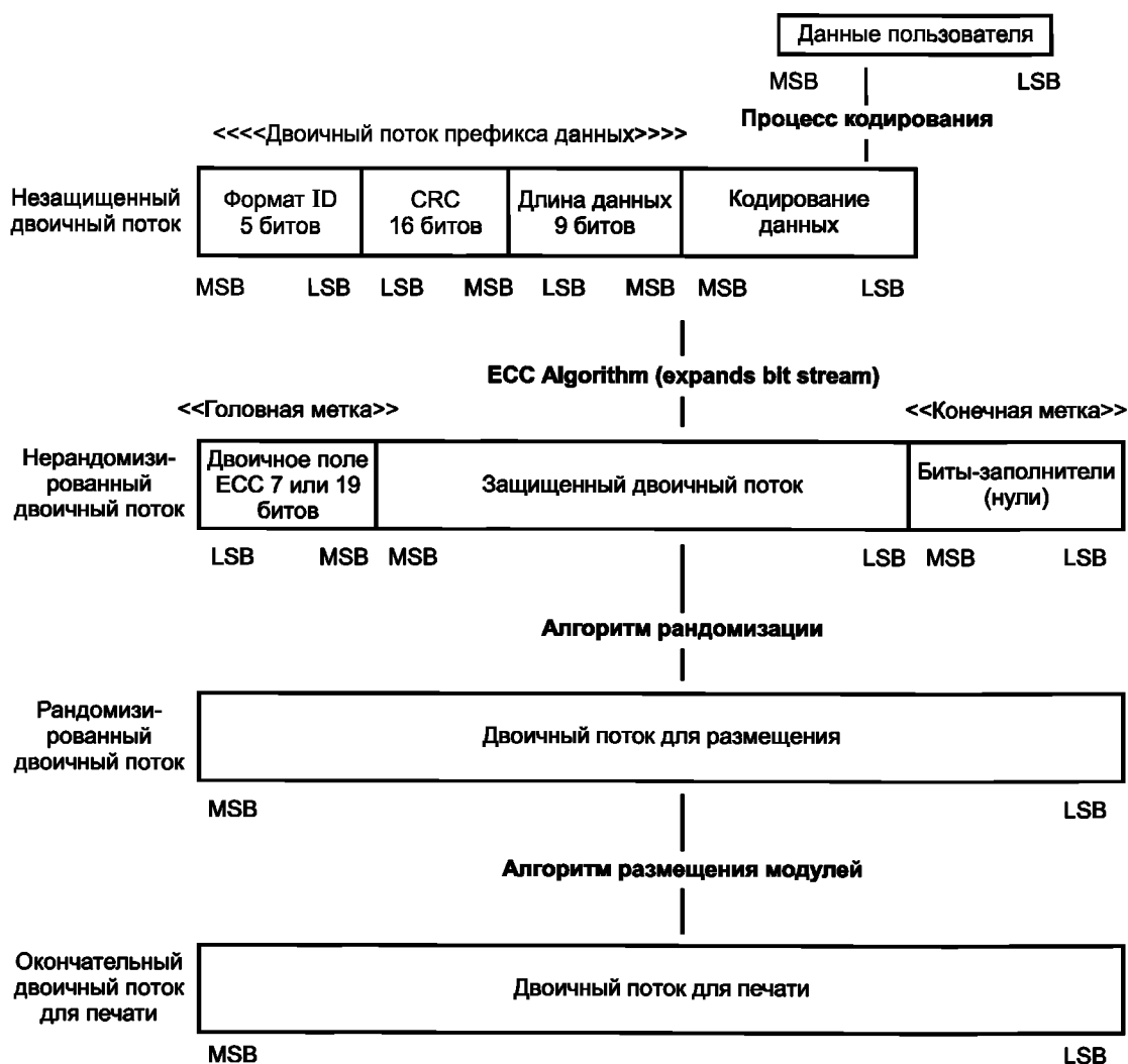
Рисунок 7 — Двоичные потоки в процессе кодирования символов версии ЕСС 000-140
