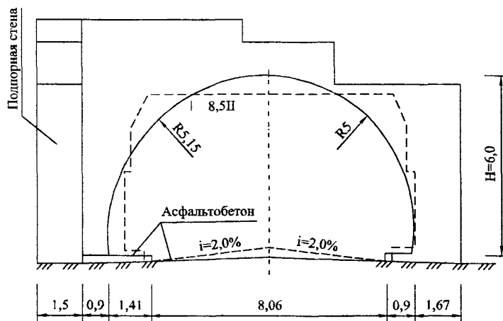
Рис. Б.1. Схема поперечного сечения тоннеля по грани южного портала (пунктиром обозначен габарит приближения строений по ГОСТ 24451)
