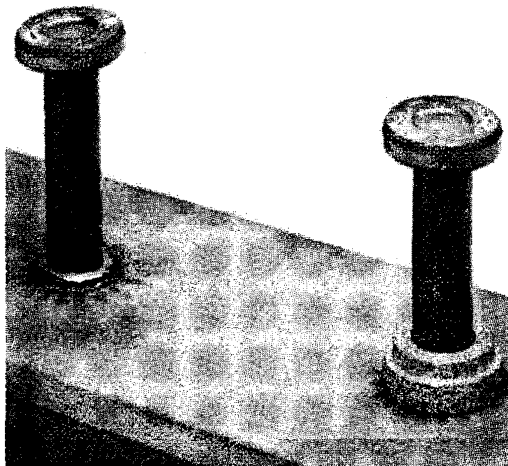
а) во время сварки б) после сварки Рисунок 4- Общий вид упоров на балке
