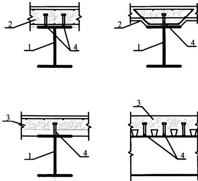
1- стальные балки 2- монолитная железобетонная плита 3- монолитная плита по профилированному стальному настилу 4- анкерный упор Рисунок 1- Сечения типовых композитных балок
