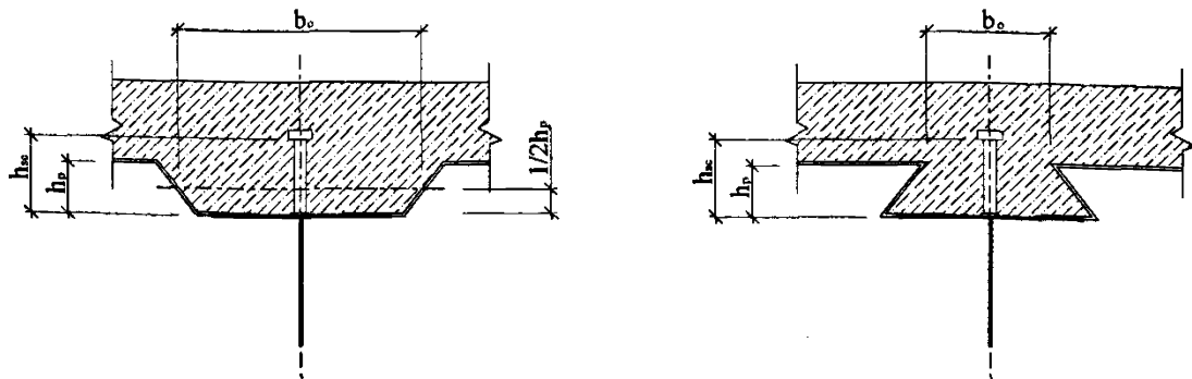
Рисунок 10- Плита с настилом, расположенным вдоль балок
