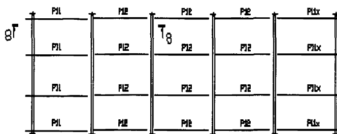
Рисунок 15 - Схема расположения стеновых однопролетных ригелей С и Z-образного сечения
