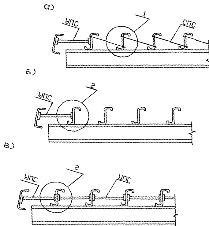
а) стержневых (СПС) б) без распорок в) угловых (УПС) Рисунок Г.1 Схемы расположения распорок между прогонами по скату
