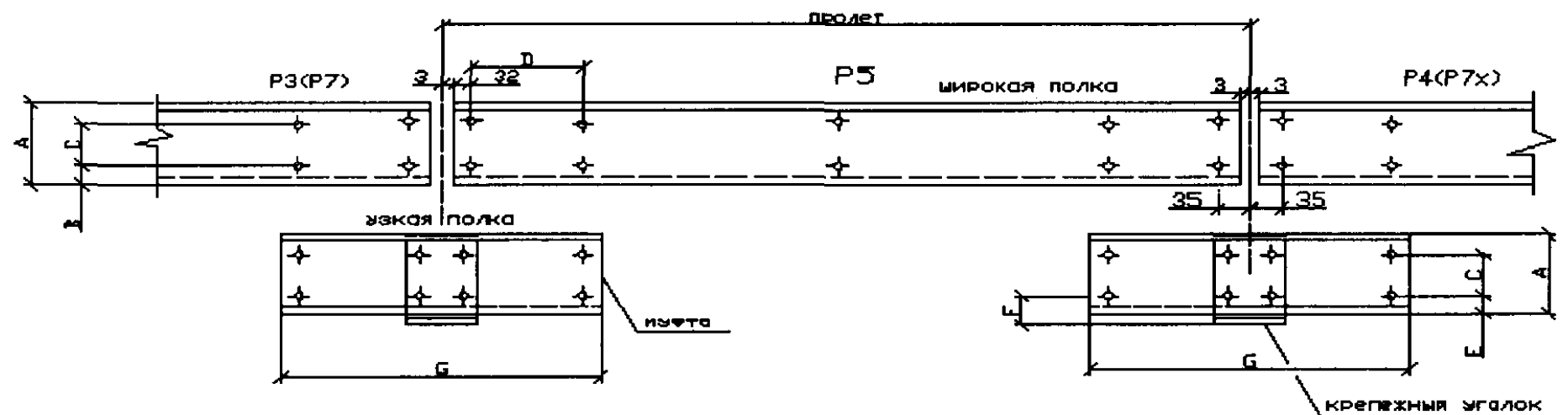
Рисунок 11 – Разрез 4-4
