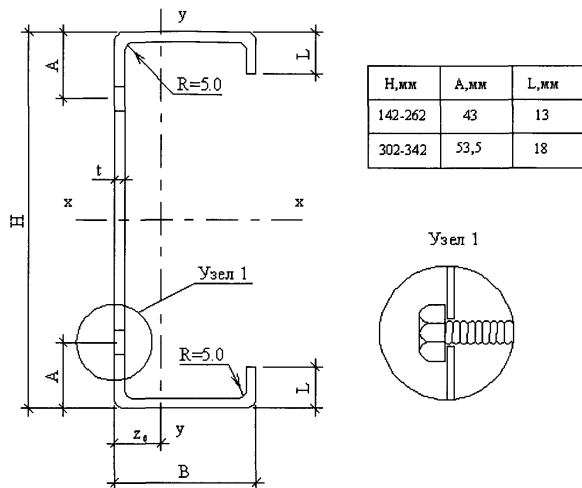
Рисунок 2-Профиль С-образного сечения
