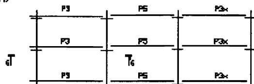
Рисунок 4-Схема расположения однопролетных прогонов Z-образного сечения
