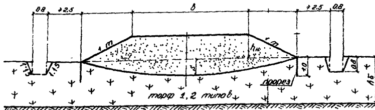
Рис. 3.2. Поперечный профиль земляного полотна на болотах I, II типов без вырезки торфа
