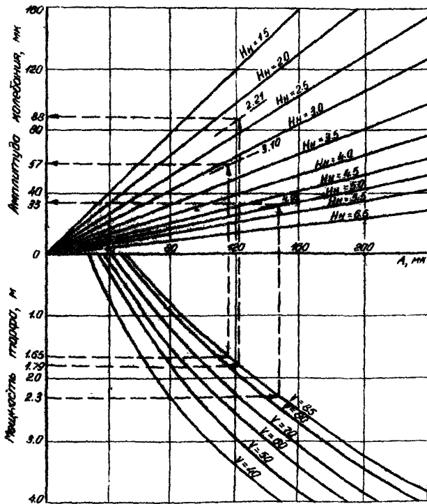
Рис. 3.14. Зависимость амплитуды колебаний от h , V_X , H_H
