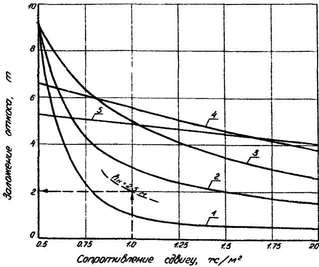
Рис. 4.12. Зависимость требуемого заложения откоса насыпи из мелкозернистого песка от сопротивления сдвигу грунта основания: 1 - h_N = 2 м; 2 - h_N = 3 м; 3 - h_N = 4 м; 4 - h_N = 8 м; 5 - h_N = 12 м
