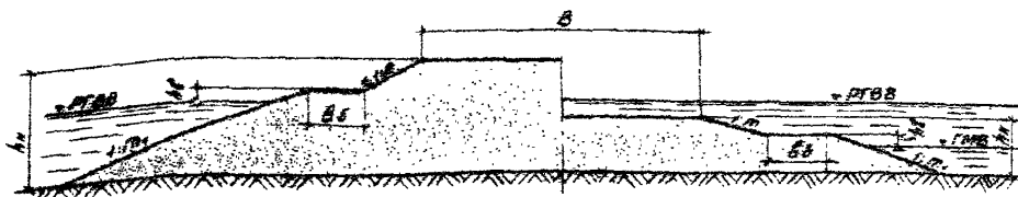
Рис. 4.5. Насыпи из песка на старицах и озерах
