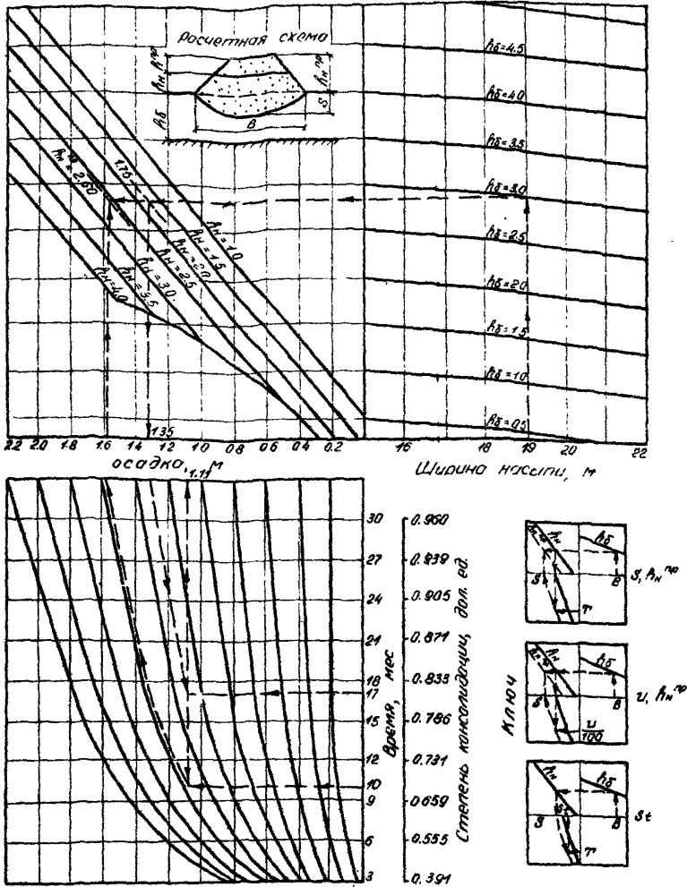
Рис. 3.10. Номограмма для определения осадки ( S ), консолидации ( U ), времени консолидации ( T ) торфяного основания и высоты временной пригрузки насыпи на болоте II типа
