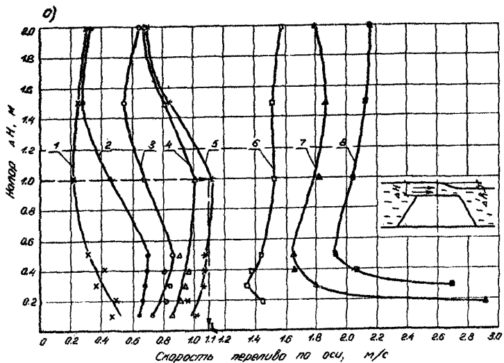
Рис. 4.14. График для определения скоростей перелива по оси (а) и на бровке (б) затопленной насадки при подпоре ( \Delta H ), равном: 1-1 см; 2-2 см; 3-3 см; 4-4 см; 5-5 см; 6-10 см; 7-15 см; 8-20 см
