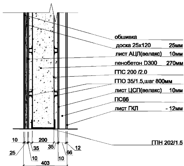
3-3 Сечение по наружной стене
