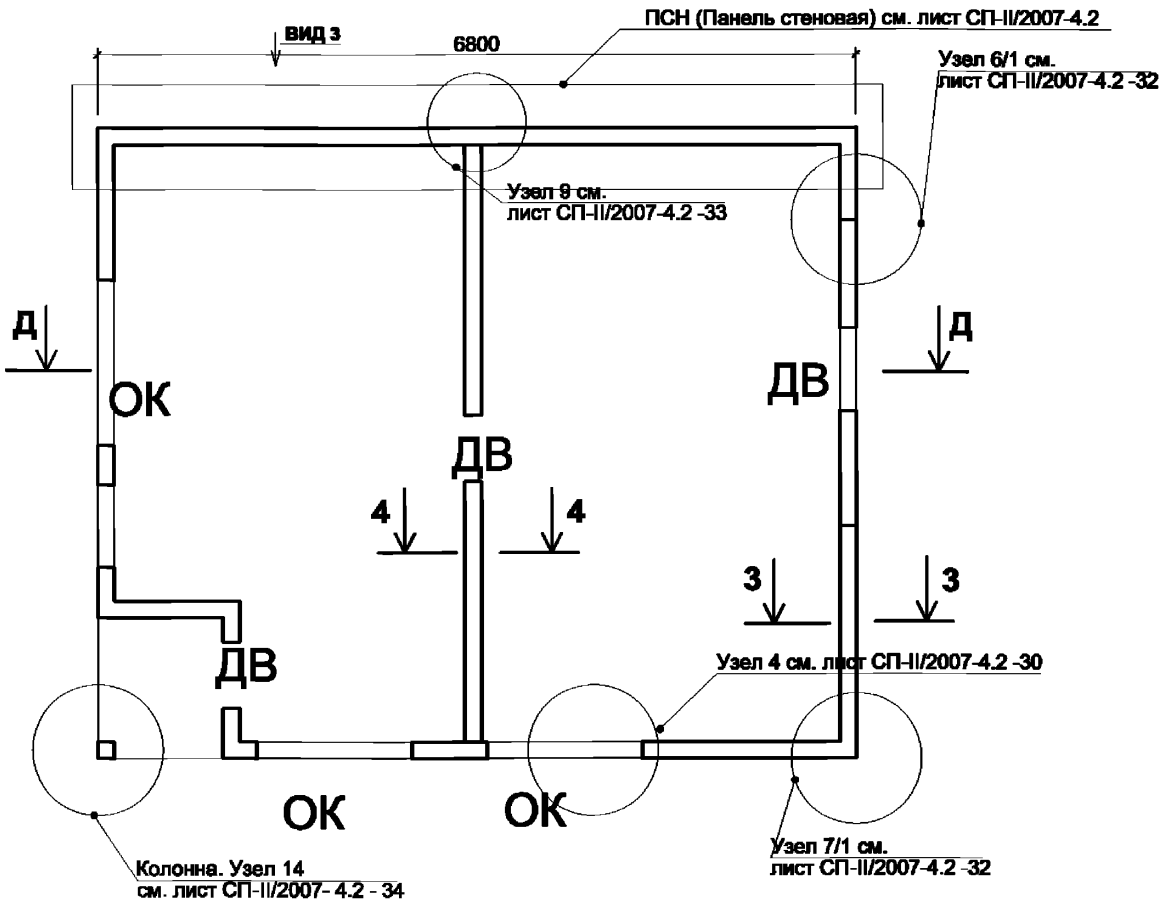
Схема плана дома
