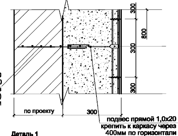
Деталь 1 для вар. 4
