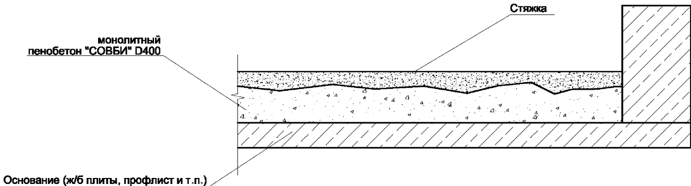
Схема заливки Вариант 2
