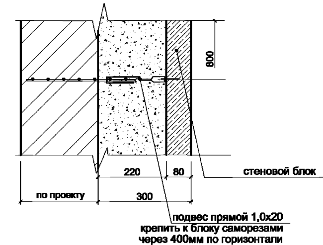
Деталь 1 Деталь фиксации каркаса и крепления листового материала вар. 1
