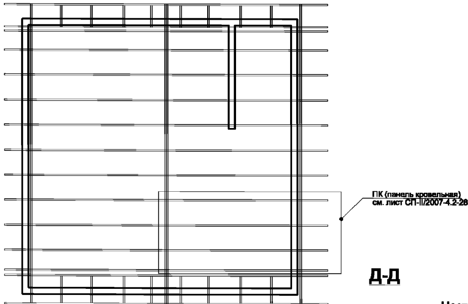
Схема расстановки стропил
