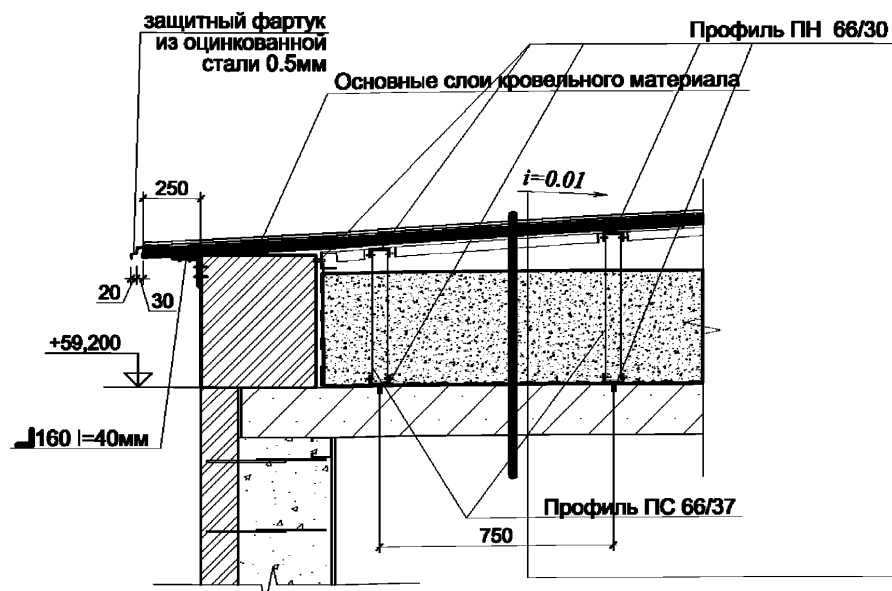
Сечение В-В для зданий без парапета
