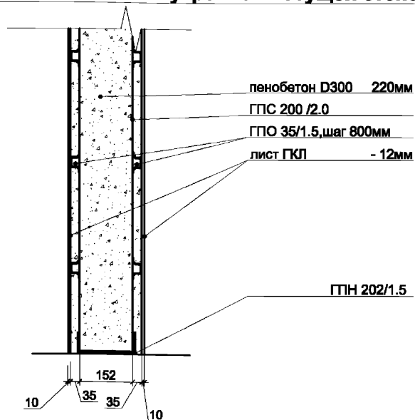
4-4 Сечение по внутренней несущей стене
