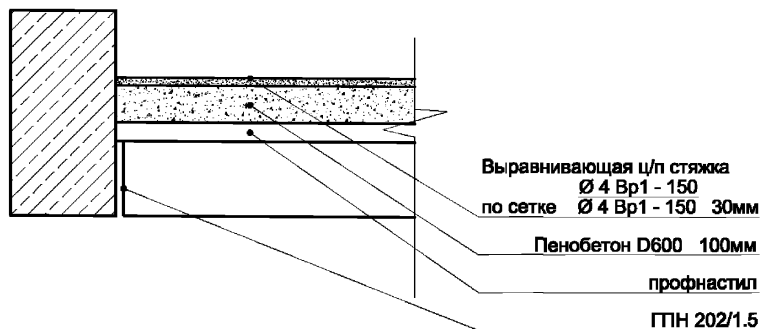
6-6 Сечение по перекрытию между 1 и 2 этажом
