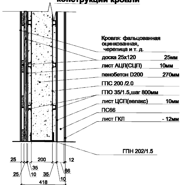
4-4 Сечение по внутренней несущей стене
