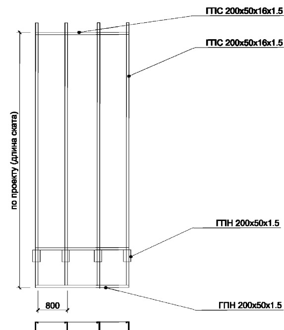
Образец кровельной панели ПК
