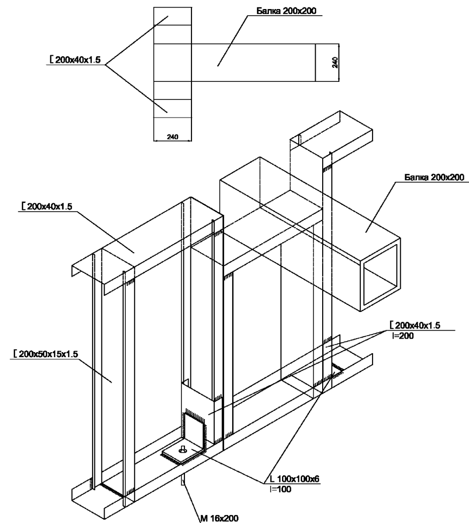
Узел крепления балки к стеновой панели
