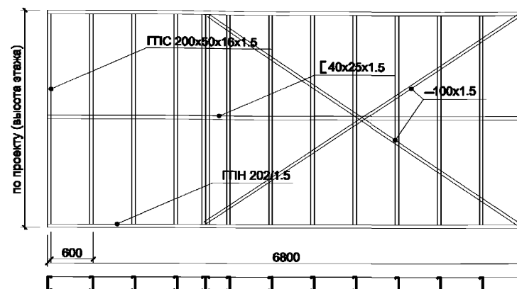
Образец стеновой панели ПСН
