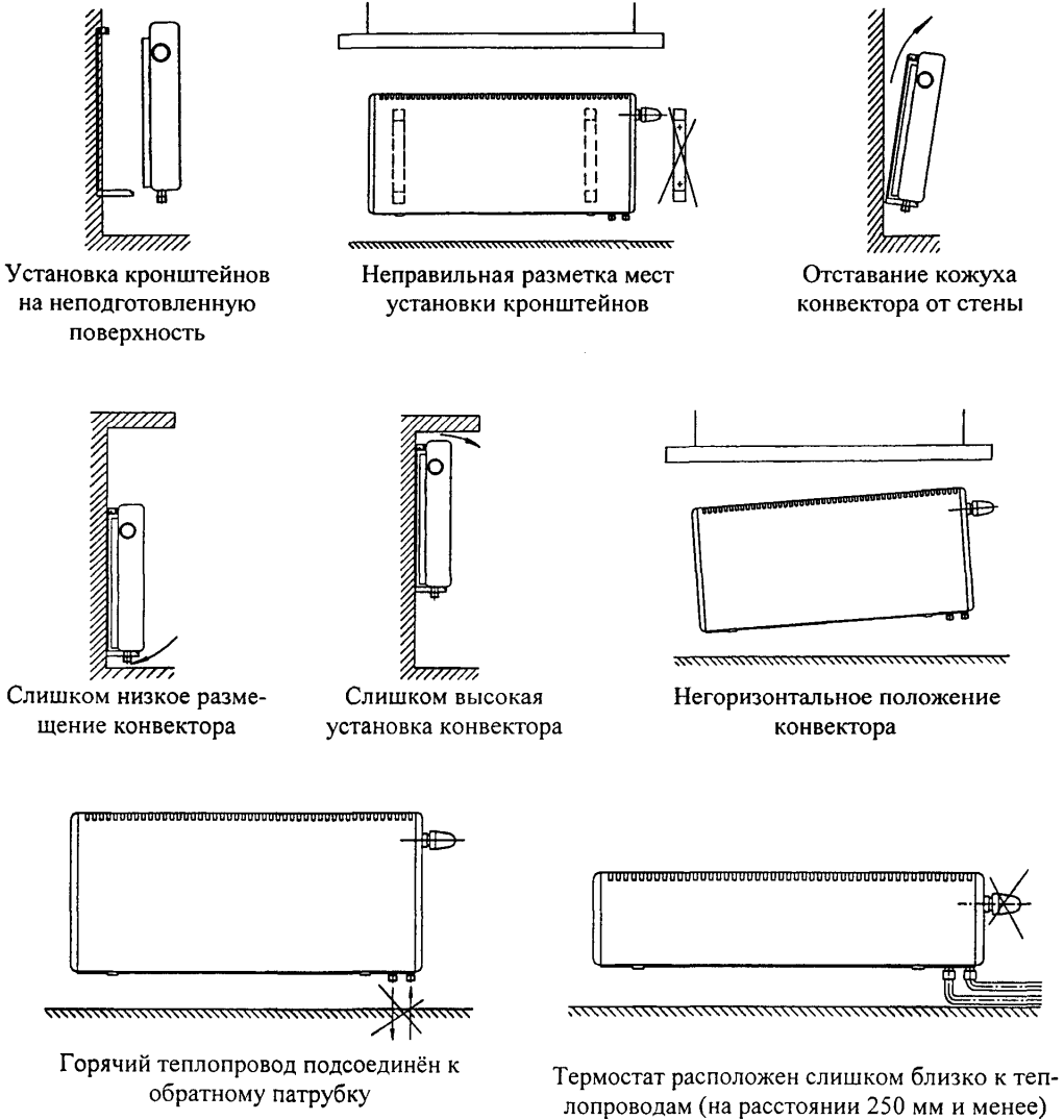
Рис. 6.2. Случаи неправильной установки конвекторов «Экотерм»
