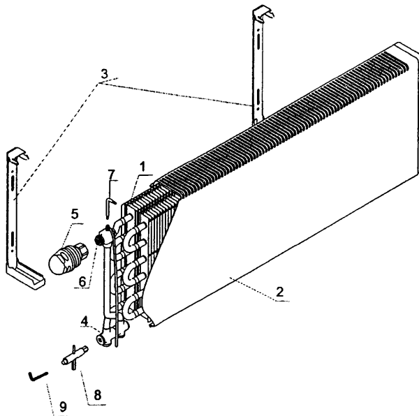
Рис. 1.4. Схема размещения основных узлов конвектора «Экотерм»
