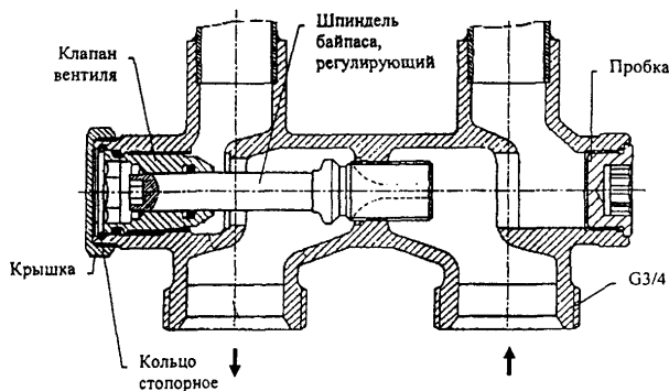
Рис. 1.5. Узел подключения конвектора «Экотерм»
