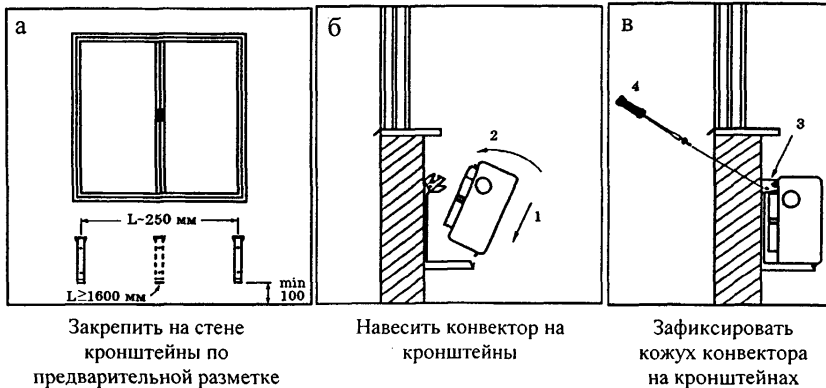
Рис. 6.1. Последовательность монтажа настенных конвекторов «Экотерм»
