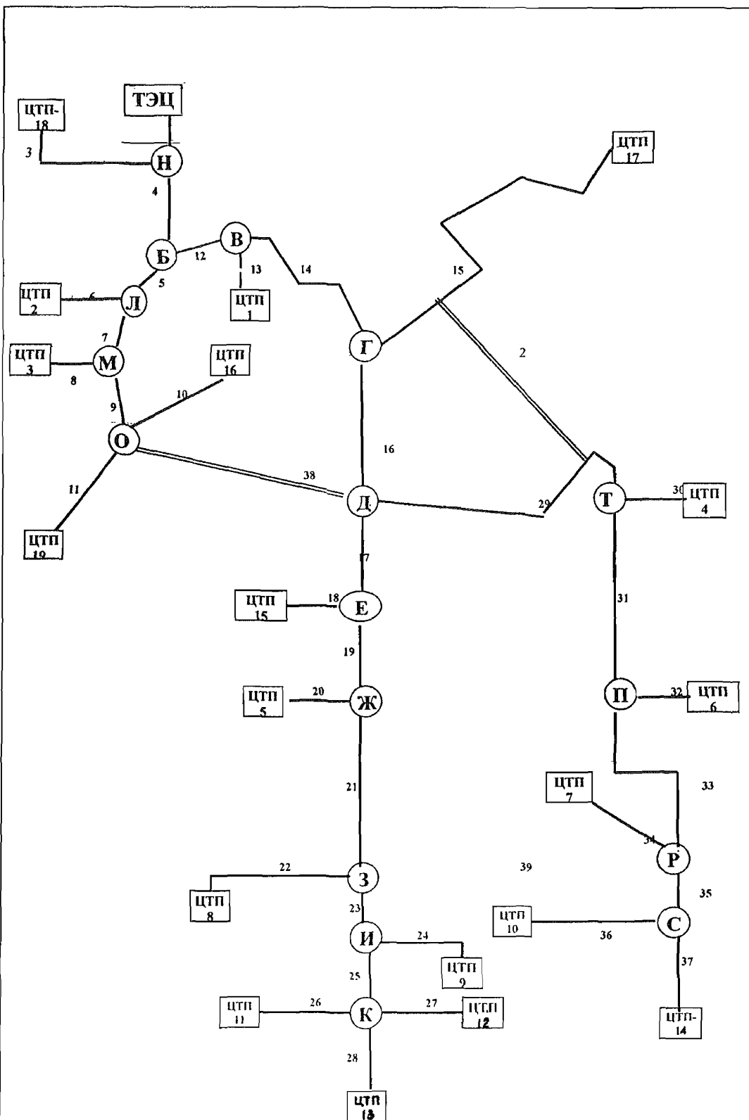
Рис. 6 Схема рекомендуемых распределительных теплопроводов г. АРТЕМЬЕВСКА: — резервный теплопровод; 1 ... 50 — участки тепловых сетей; Н — насосная; ТЭЦ — теплоэлектроцентраль; ЦТП — центральные тепловые пункты;
