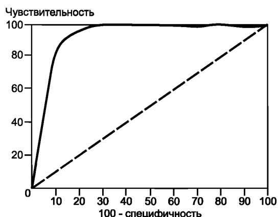
Рисунок 3 — ROC-кривая
