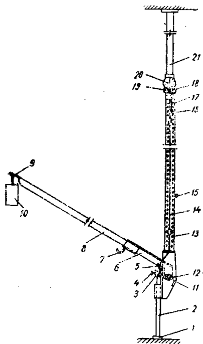
Рис. 1 Схема деформатора
