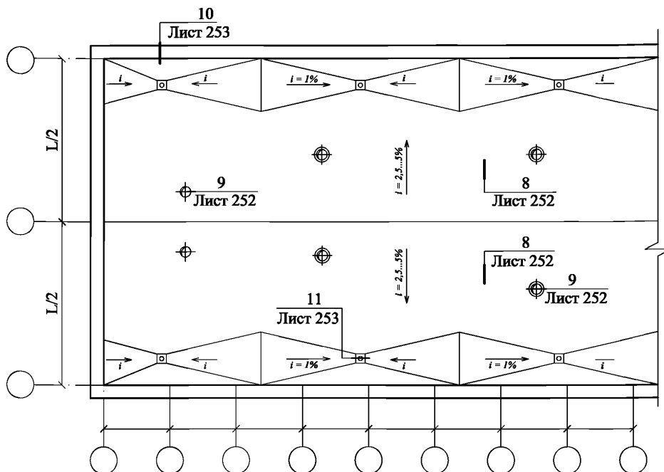
План кровли
