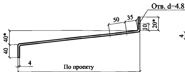
КОСТЫЛЬ K2
