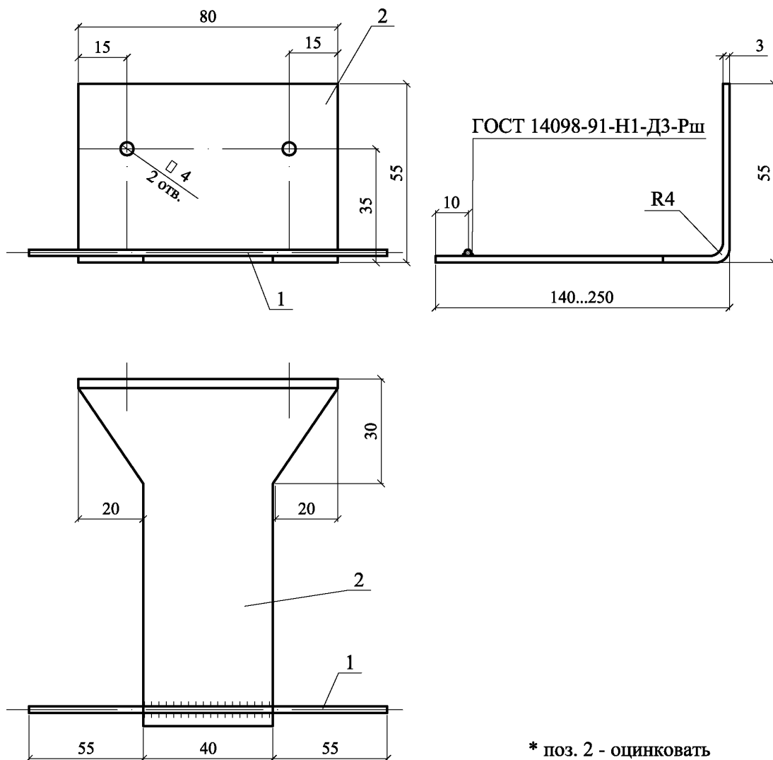
АНКЕР А1
