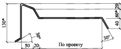
КОСТЫЛЬ K1
