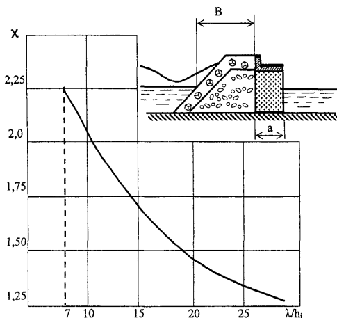
Рисунок 5.8 - График для определения коэффициента \chi = f(\bar{\lambda} / h)
