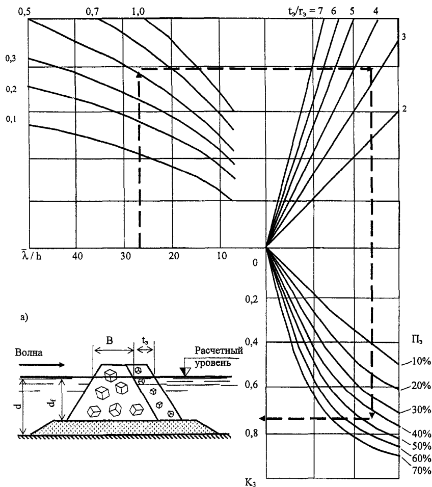
Рисунок 5.7 - Схема (а) и графики (б) для определения коэффициента затухания волн K_3 при наличии тылового экрана в набросном сооружении
