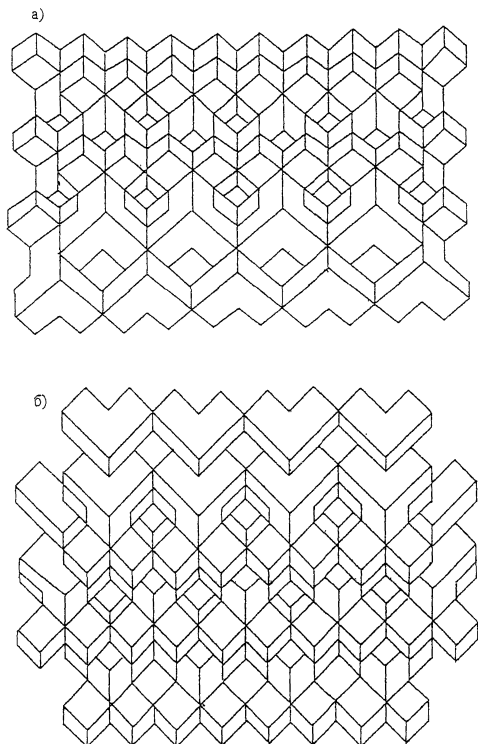
Рисунок Б.5 – Схемы двухслойной укладки пентапонов
