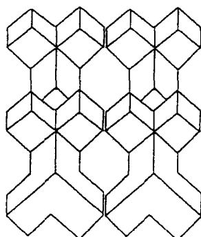
Рисунок Б.4 – Схемы однослойной укладки пентаподов
