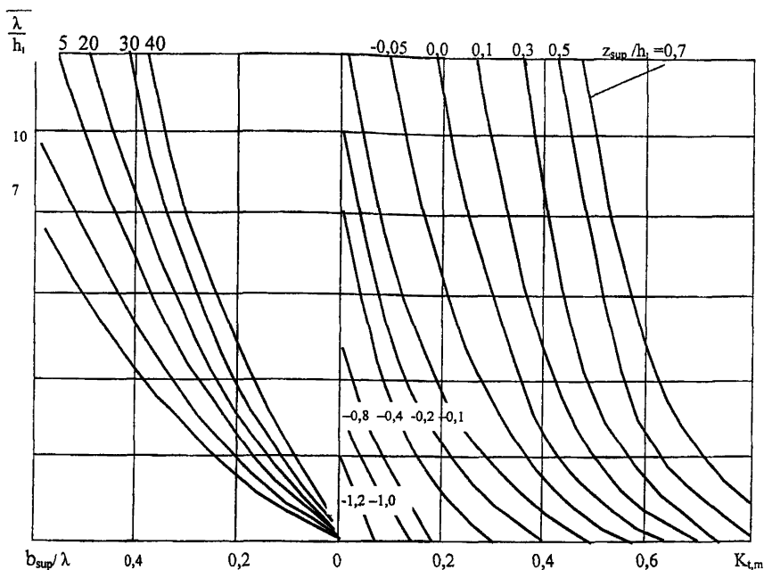
Рисунок 5.5 - Схема (а) и графики (б) для определения коэффициентов прохождения K_{т,м} ветровых волн через верх набросного сооружения неполного профиля с ядром из несортированного камня
