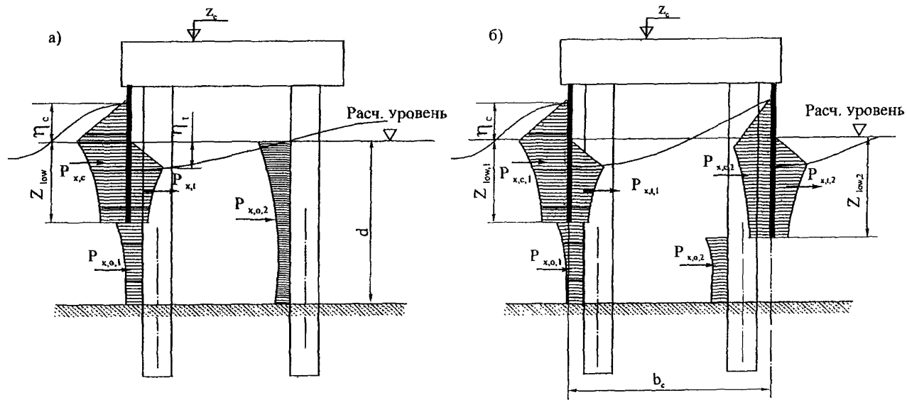
Рисунок 6.4 - Эпюры волнового давления на элементы сквозных ограждающих сооружений в виде одиночного экрана (а) и двух вертикальных экранов (б)
