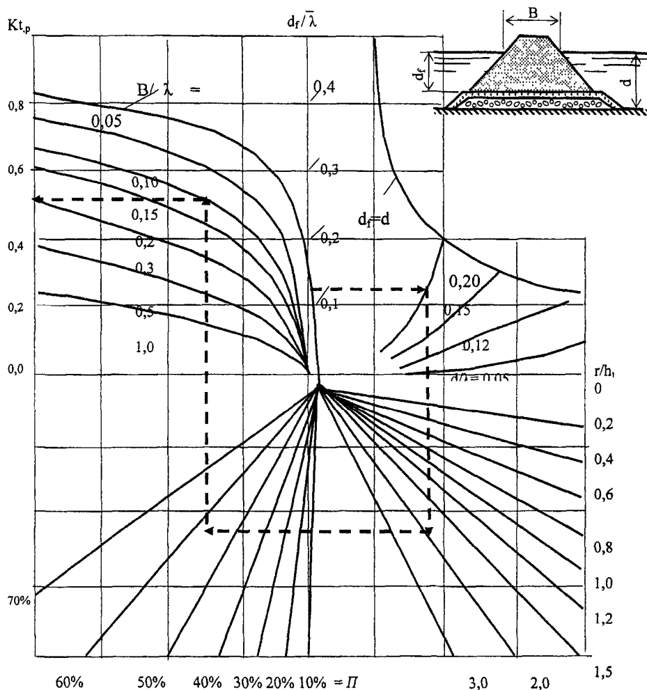
Рисунок 5.6 - Графики для определения коэффициентов прохождения K_{t,p} сквозь однородное сооружение из наброски крупного камня, фасонных блоков или массивов
