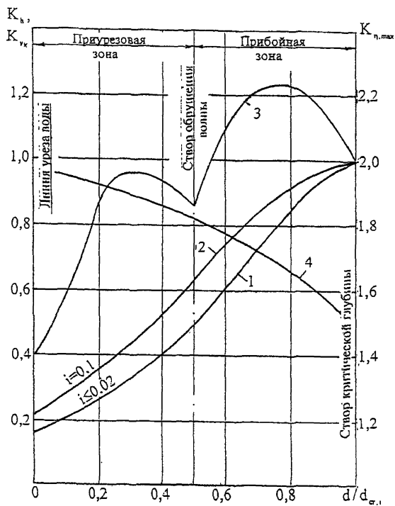
Рисунок А.3 - Графики для определения коэффициентов K_k (1 и 2), K_{\eta, \max} (3) и K_{\eta, \max} (4)
