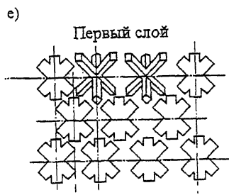
Рисунок Б.2 – Схемы укладки гексалегов на откосе
