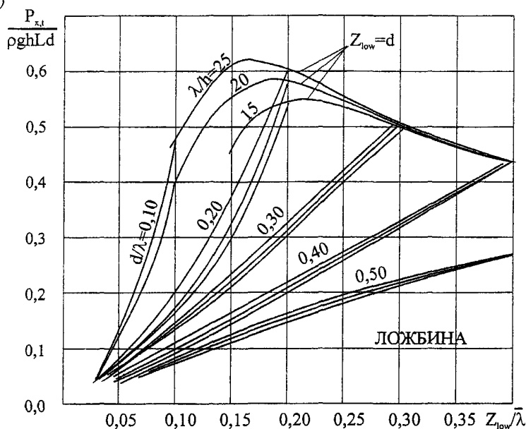
а – при подходе гребня волны; б – при подходе ложбины волны Рисунок 6.3 – Графики для определения суммарной волновой нагрузки на сплошной экран при подходе гребня (а) и ложбины (б) волны
