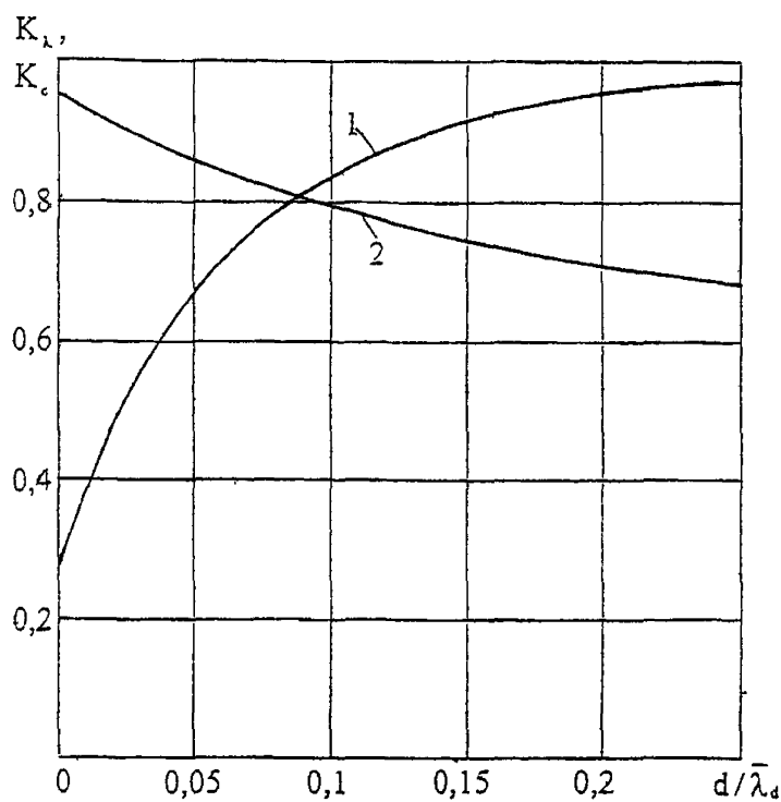
Рисунок А.2 - Графики для определения коэффициентов K_\lambda (1) и K_\epsilon (2)
