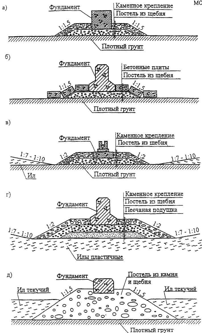
Рисунок 7.2 – Схемы конструкций подводных стендов
