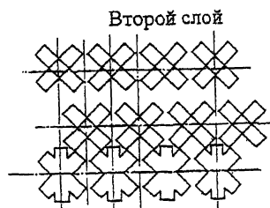
Рисунок Б.2 – Схемы укладки гексалегов на откосе
