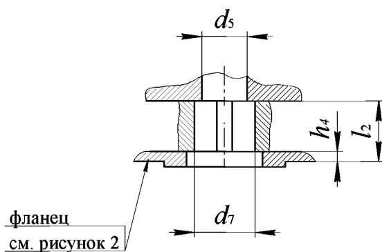
Рисунок 6 – Ведущие подвижные детали группы В
