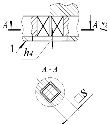
1 – поверхность взаимодействия
