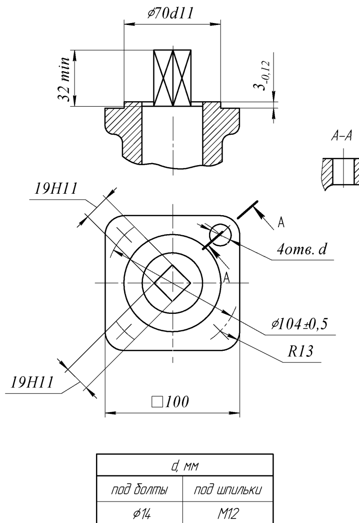
Рисунок А.6 – Ответное присоединение трубопроводной арматуры типа АЧ
