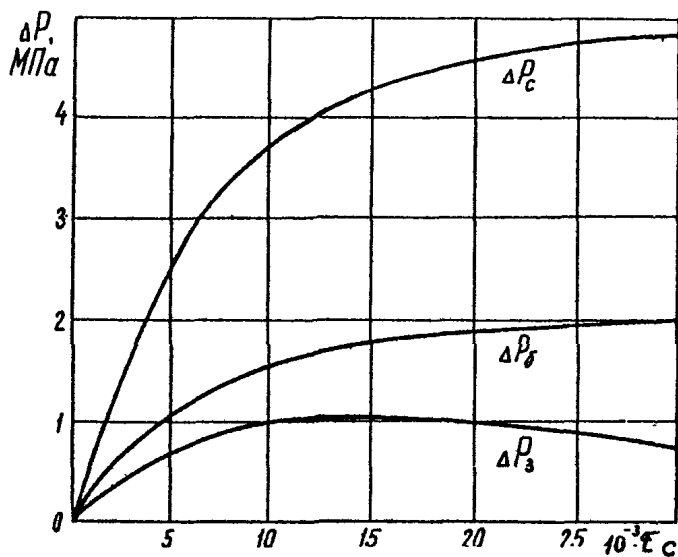
Рис. 2.36. Кривые восстановления затрубного ( \Delta P_s ) буферного ( \Delta P_f ) и забойного давления ( \Delta P_c ) нефтяной скважины
