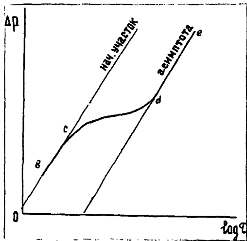
Рис. 2.13. Преобразованная кривая восстановления давления, характерная для трещиновато-пористого пласта.
