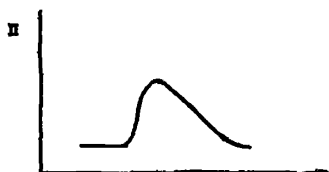
Рис. 4.3. Типичная озонграмма элюата нефти.
