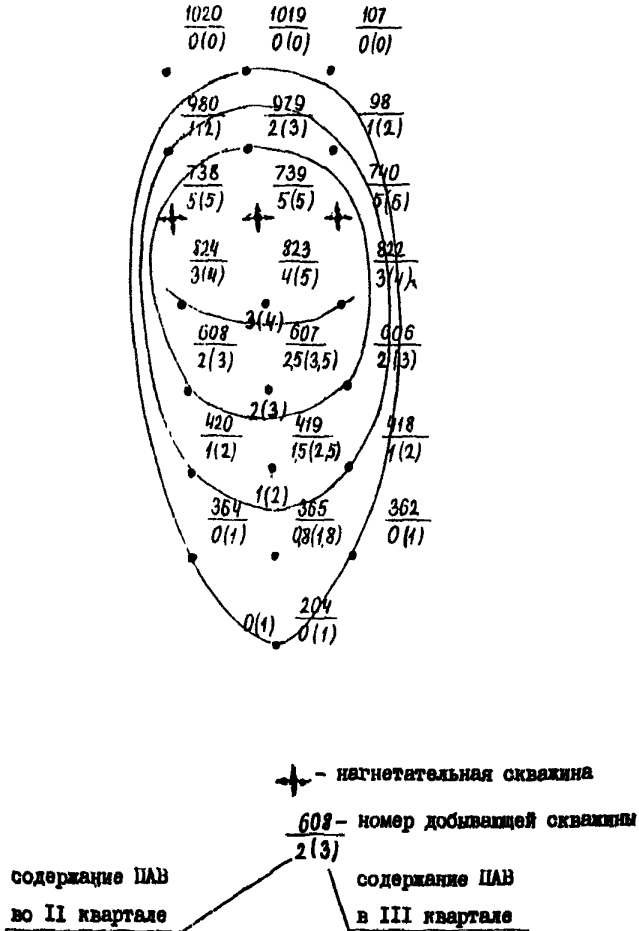
Рис.5.II Карта распределения содержания ПАВ (% мас.) в извлекаемой воде по состоянию на II и III кварталы 1988 г.
