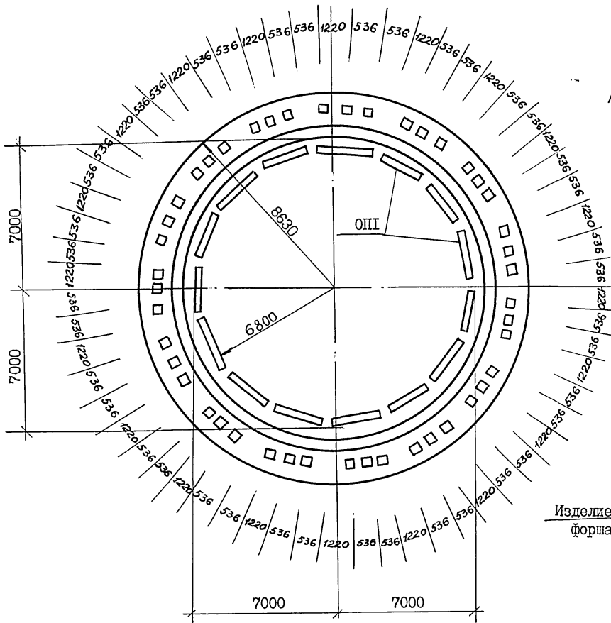
Схема расположения опорных блоков и форшахты при опускном способе
