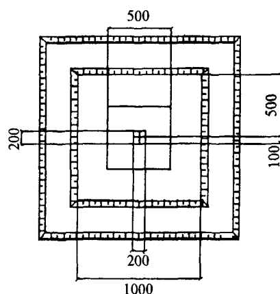
Вид А
