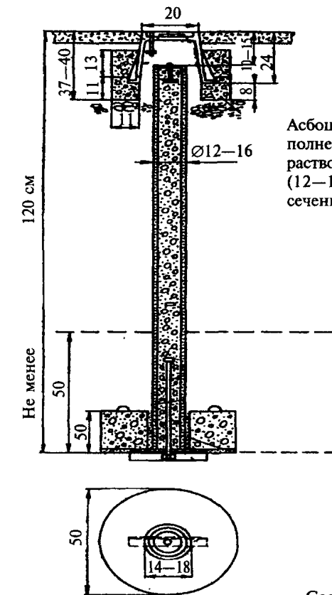
Бетонный якорь Ø50 см
