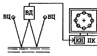
Рис.2. Схема видеоуровнемера
