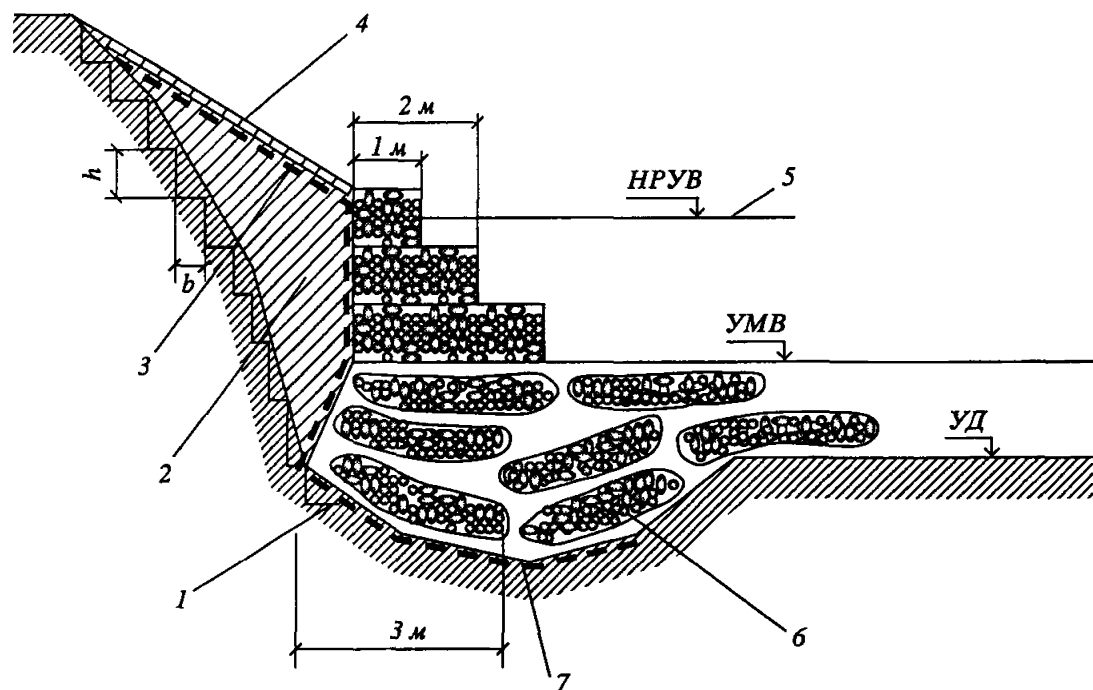
Рис. 4.15. Проектное положение конструкции:
