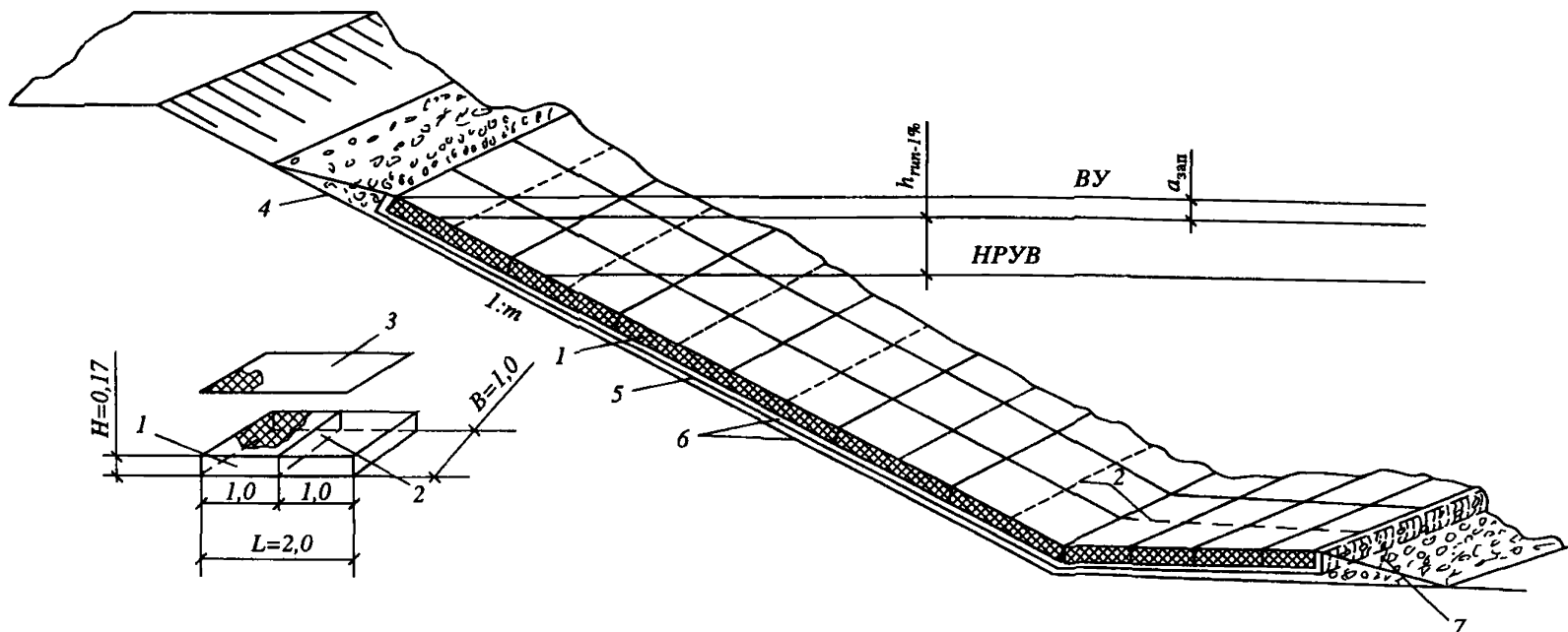
Лист. 1. Однослойная защита из габийонных тюфяков (матрасов Рено) МД1
