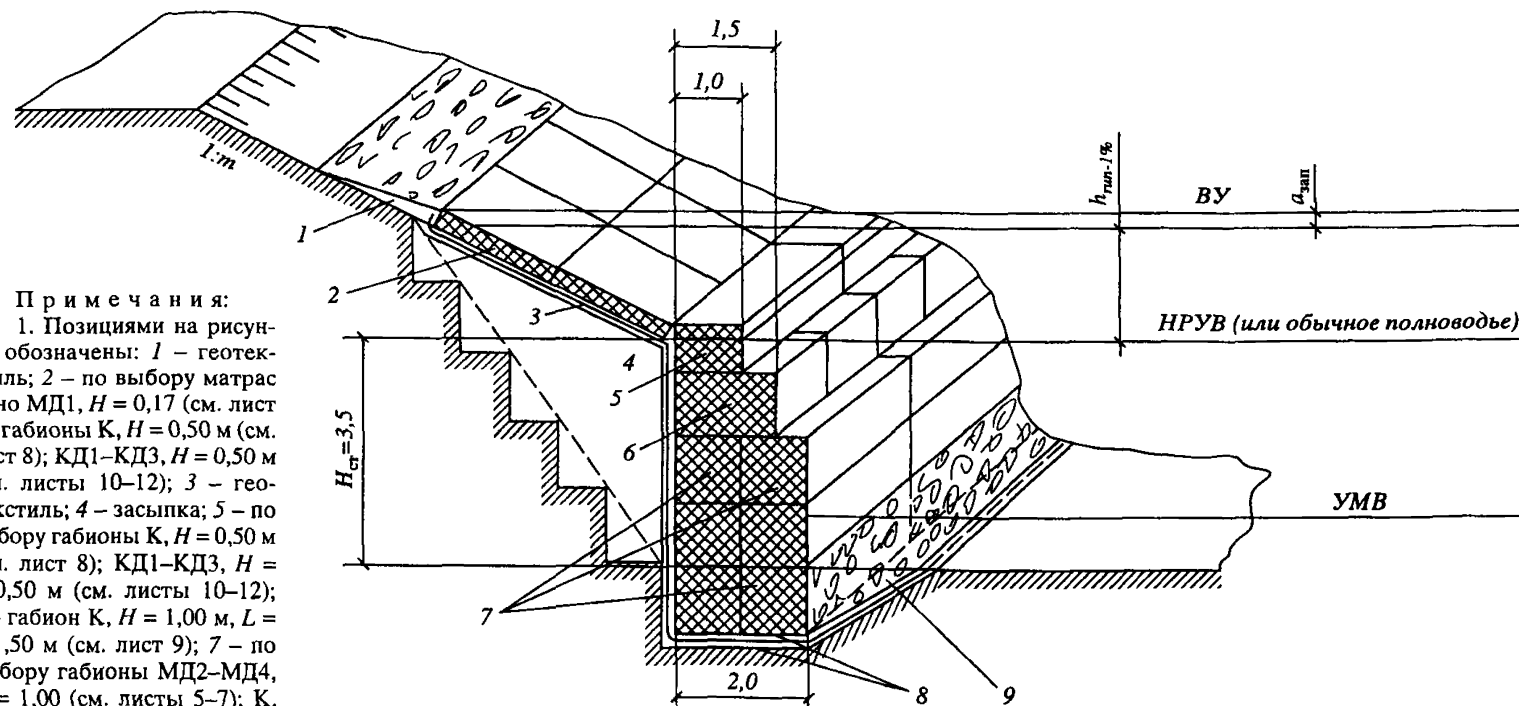
Лист 24. Комбинированная защита с гравитационной габионной стеной, H_{\text{ст}} = 3,5 м (вариант I)
