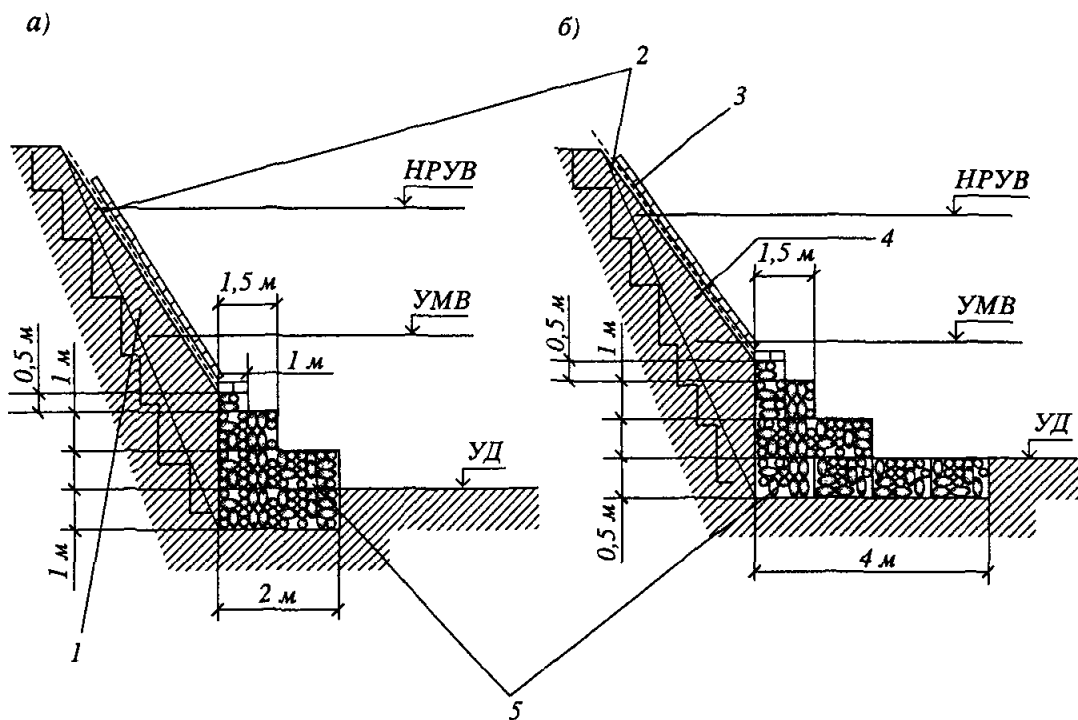
Рис. 4.19. Проектное положение габионных защит:
