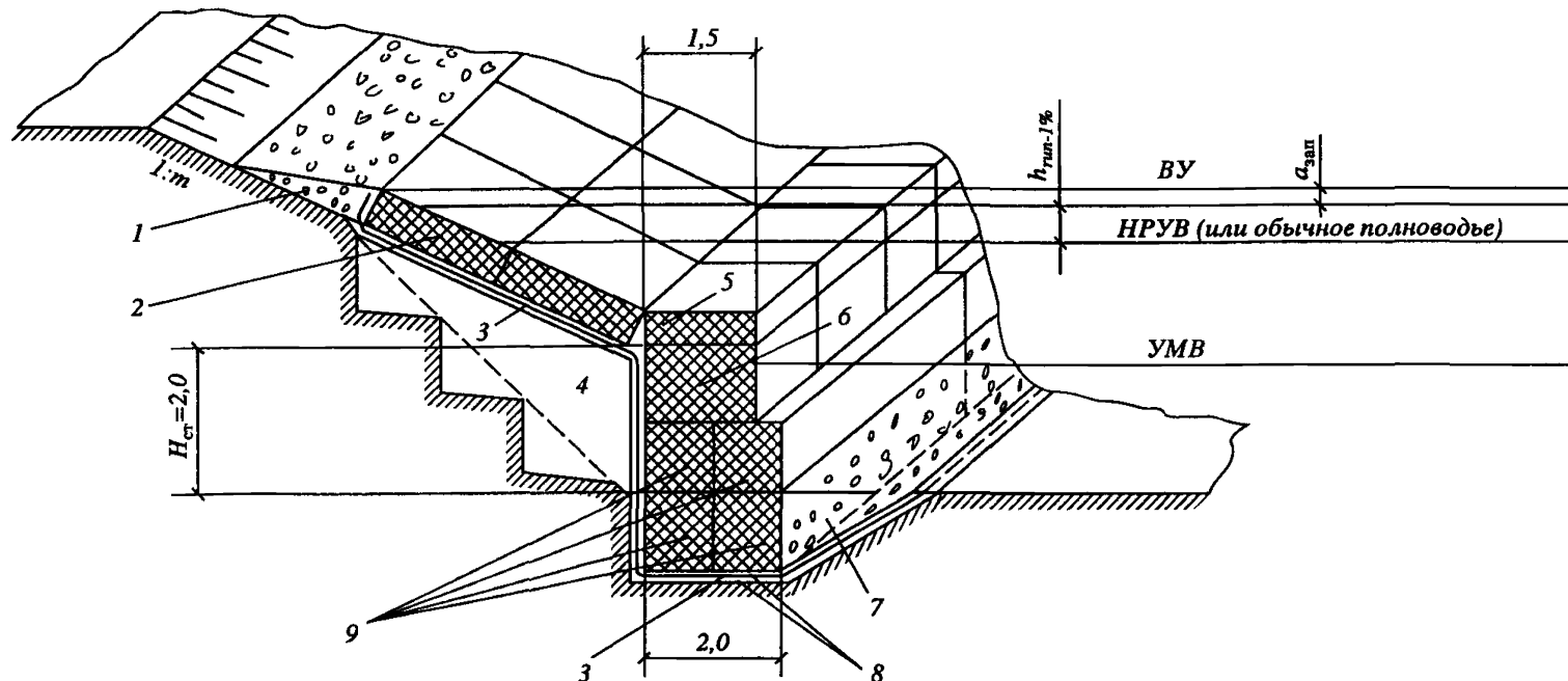
Лист 18. Комбинированная защита с гравитационной габионной стеной, H_{\text{ст}} = 2,0 м (вариант I)
