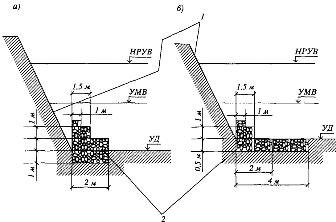
Рис. 4.18. Схема установки блоков габиона стены:
