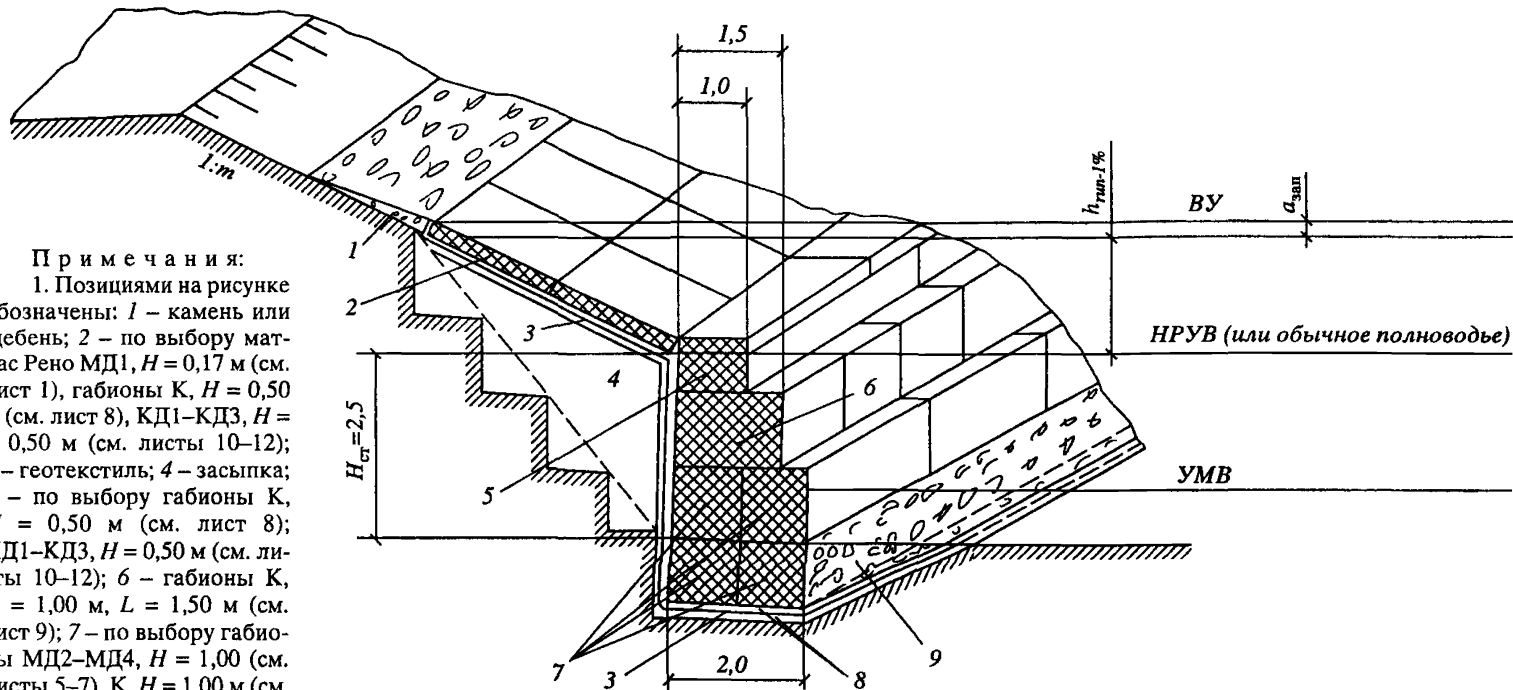
Лист 20. Комбинированная защита с гравитационной габионной стеной, H_{ст} = 2,5 м (вариант I)
