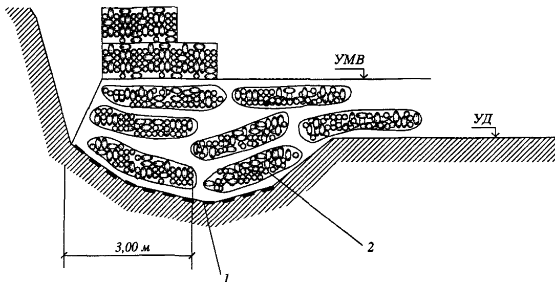
Рис. 4.14. Схема монтажа последующих коробчатых габионов:
