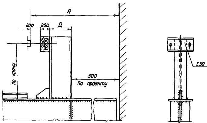
Рис.58. Схема размещения концевых упоров для мостовых кранов
