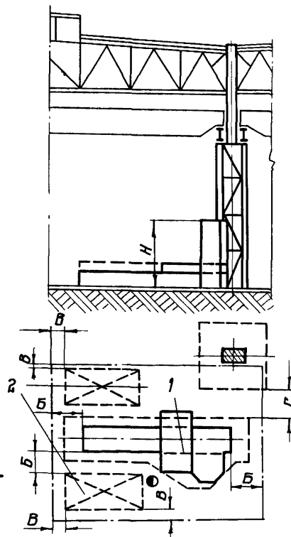
Рис.22. Размещение продольно-строгального станка в поперечном пролете: I - станок продольно-строгальный; 2 - место складирования
