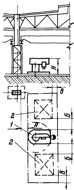
Рис. 25. Размещение радиально-сверлильного станка в поперечном пролете: 1 - станок; 2 - место складирования
