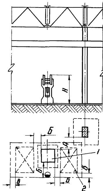
Рис. I4. Размещение винтового прессы в продольном пролете: I - пресс; 2 - место складирования
