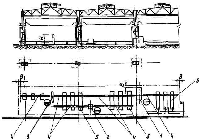
Рис.31. Размещение линии обработки швеллеров и балок: 1 - станок отрезной; 2 - станок горизонтально-свер- лильный; 3 - станок вертикально-сверильный; 4 - роль- ганг; 5 - транспортер поперечный
