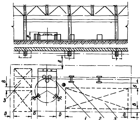
Рис.8. Размещение сортогибочной машины в продольном пролете: 1 - машина; 2 - козелок переставной; 3 - место складирования
