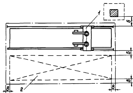
Рис. 39. Размещение радиально-сверлильного станка (передвижного) в поперечном пролете: 1 - станок; 2 - место складирования
