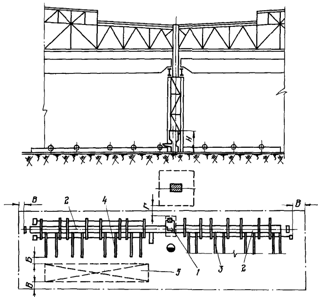
Рис.15. Размещение дыропробивного прессы в поточной линии: 1 - пресс; 2 - ролик; 3 - транспортер поперечный; 4 - сбрасыватель; 5 - место складирования
