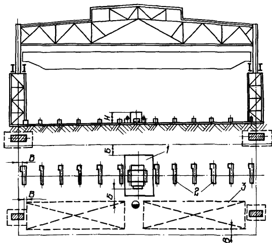
Рис.35. Размещение машины для правки гибовидности сварных двутавровых балок в поперечном пролете: 1 - станок; 2 - ролики опорные; 3 - место складирования
