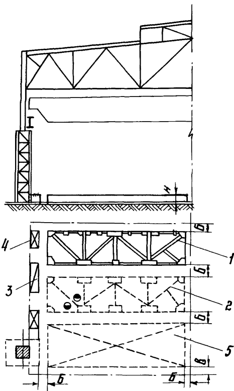
Рис.48. Размещение участка для сборки конструкций в поперечном пролете: I - сборка окончательная; 2 - кондуктор для сборки; 3 - ящик для инструмента; 4 - трансформатор сварочный; 5 - место складирования
