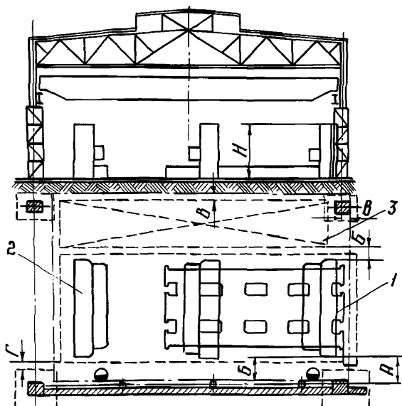
Рис. 36. Размещение двухстороннего торцефрезерного станка в поперечном пролете: 1 - подвижная часть станка с фрезой; 2 - неподвижная часть станка с фрезой; 3 - место складирования
