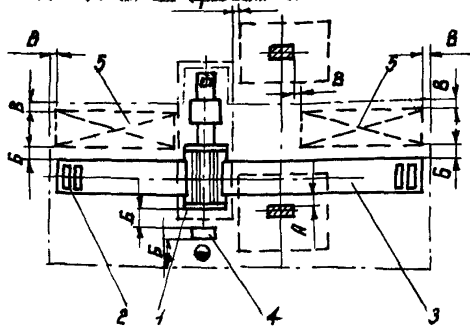
Рис. 1. Размещение листопрямляющей машины вне поточной линии: 1 - вальцы; 2 - ролик подающий; 3 - ролик приемный; 4 - пульт управления; 5 - место складирования
