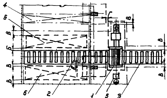
Рис. 2. Размещение листопрямляющей машины в поточной линии: 1 - вальцы; 2 - ролик подающий; 3 - ролик приемный; 4 - укладчик магнитный; 5 - пульт управления; 6 - место складирования
