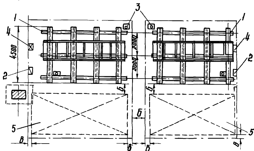
Рис. 50. Размещение стенда для сварки из козелков в поперечном пролете: 1 - козелок; 2 - ящик для инструмента; 3 - полуавтомат сварочный; 4 - источник питания; 5 - место складирования
