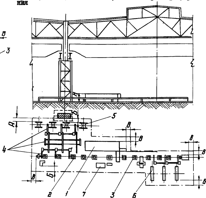
Рис. 28. Размещение автомата фирмы "Пайком" для газовой фасонной резки труб в поточной линии:
