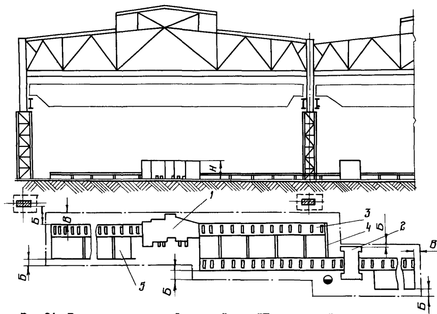
Рис.34. Размещение поточной линии фирмы "Пединггауз" для обработки швеллеров и балок: 1 - станок сверлильный агрегатный; 2 - станок отрезной; 3 - рольганг; 4 - устройство для поперечной передачи; 5 - стеллаж
