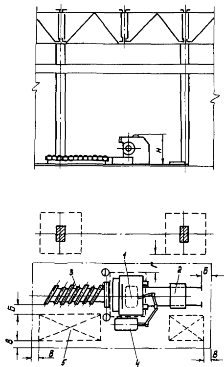
Рис.19. Размещение гильотинных ножиц при поперечной резке листа:
