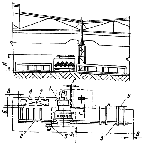
Рис. 3. Размещение сортоправильной машины в поточной линии: 1 - валцы сортоправильные; 2-рольганг подающий; 3 - рольганг приемный; 4 - стеллаж загрузочный; 5 - транспортер поперечный; 6 - пульт управления; 7 - место складирования
