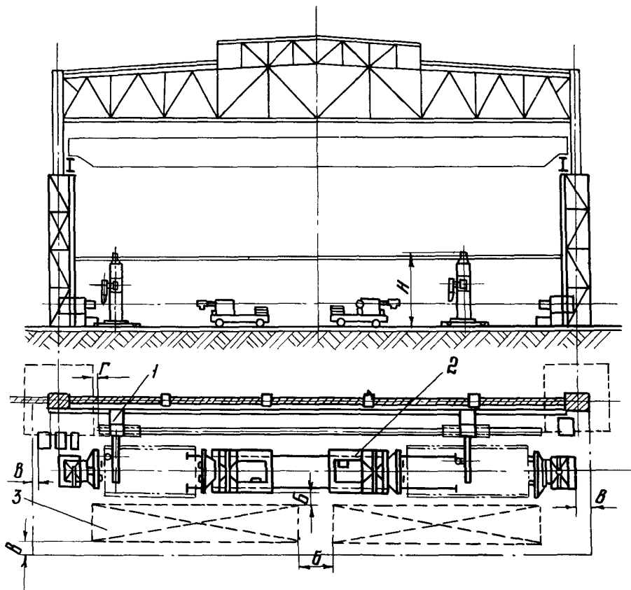
Рис.41. Размещение участка автоматической сварки с велосипедной тележкой: 1 - тележка велосипедная; 2 - кантователь двухколесный; 3 - место складирования
