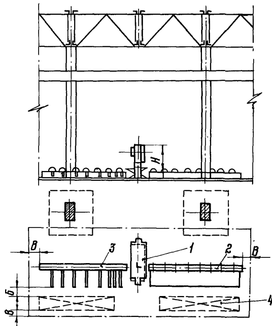
Рис. I7. Размещение комбинированных пресс-ножиц в продольном пролете: 1 - пресс-ножицы; 2 - ролик подающий; 3 - ролик приемный; 4 - место складирования
