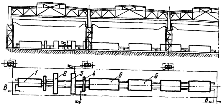
Рис.40. Размещение поточной линии для сборки и сварки подкрановых балок: 1 - кондуктор; 2 - кантователь; 3 - кантователь; 4 - траверса; 5 - кондуктор; 6 - подъемник
