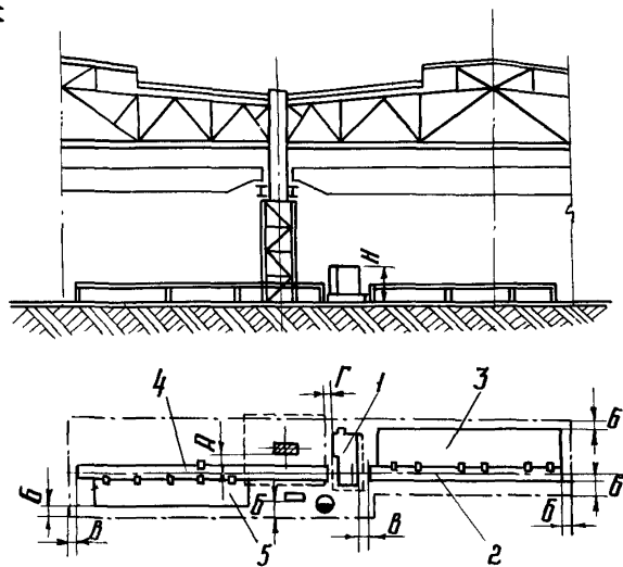
Рис. 24. Размещение фрезерно-отрезного станка для резки бабок: 1 - станок отрезной; 2 - ролик подающий; 3 - стеллаж загрузочный; 4 - ролик приемный; 5 - стеллаж для деталей
