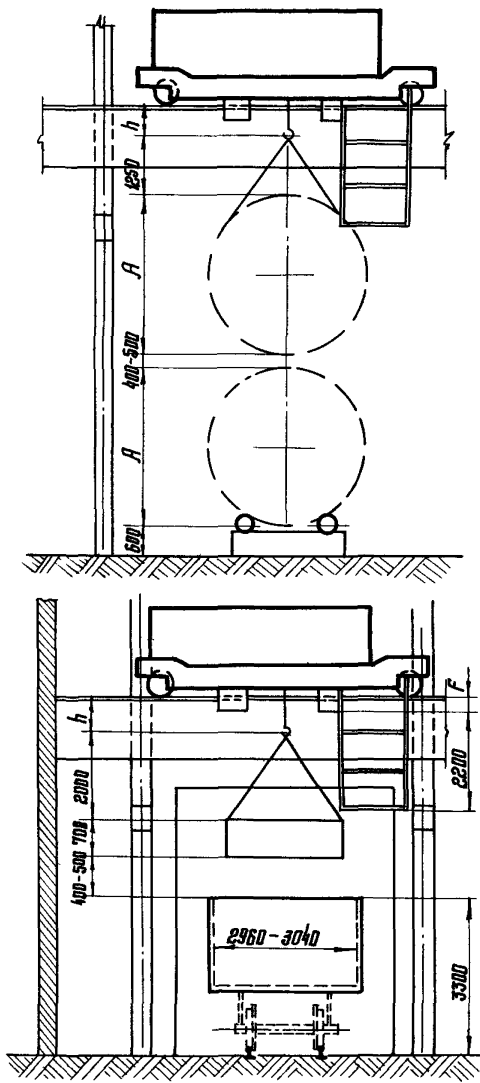
Рис. 55. Схема размещения мостового крана над железнодорожной платформой
