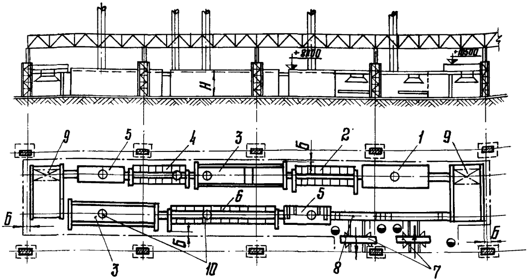
Рис.52. Размещение поточной линии окраски конструкций методом облива длиной до 12 м:
