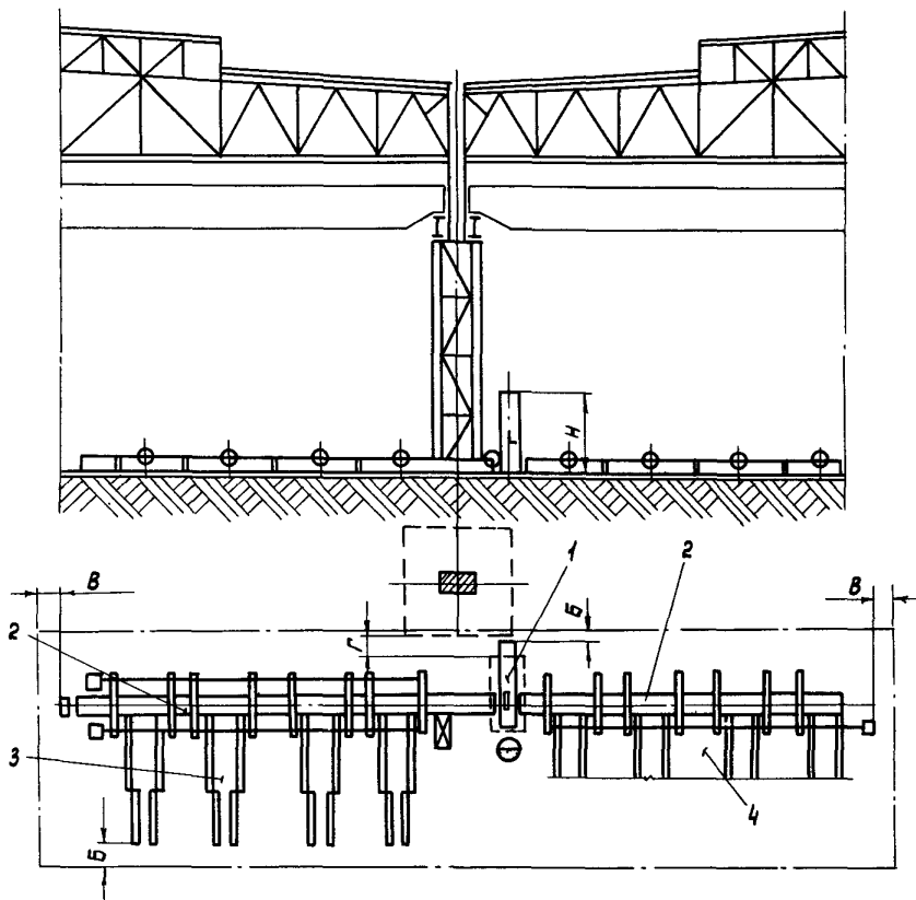
Рис.18. Размещение ножниц для резки профильного проката в поточной линии: 1 - ножницы; 2 - рольганг; 3 - стеллаж для проката; 4 - накопитель
