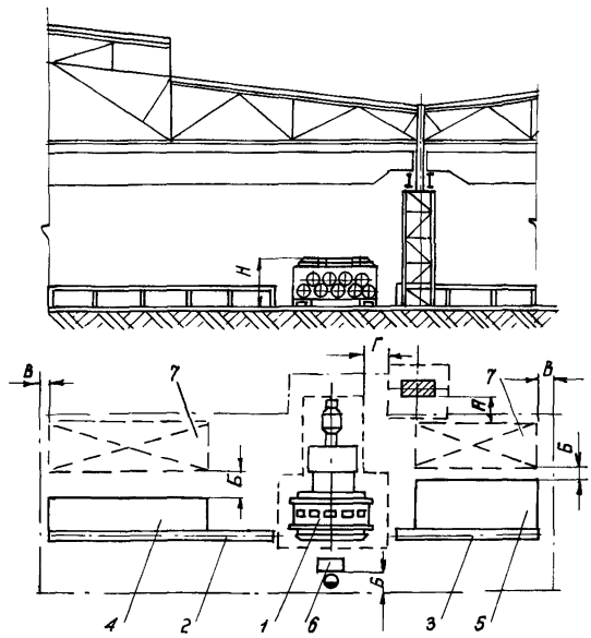
Рис. 4. Размещение сортоправильной машины вне поточной линии: 1 - валцы сортоправильные; 2 - рольганг подающий; 3 - рольганг приемный; 4 - стеллаж загрузочный; 5 - стеллаж приемный; 6 - пульт управления; 7 - место складирования
