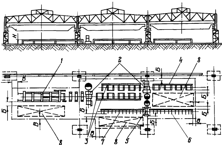
Рис.44. Размещение поточной линии сборки, сварки и резки стержней двутаврового сечения: 1 - стол для сборки стержней; 2 - агрегат сварочный; 3 - ролик и кантователь; 4 - ролик конечный; 5 - машина для кислородной резки трехрежковая; 6 - ролик подающий; 7 - ролик приемный; 8 - место складирования
