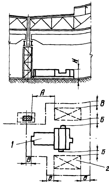
Рис.23. Размещение поперечно-строгального станка в поперечном пролете: 1 - станок поперечно-строгальный; 2 - место складирования
