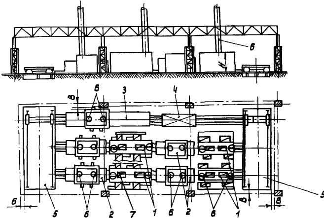
Рис.53. Размещение поточной линии окраски конструкций методом распыления:
