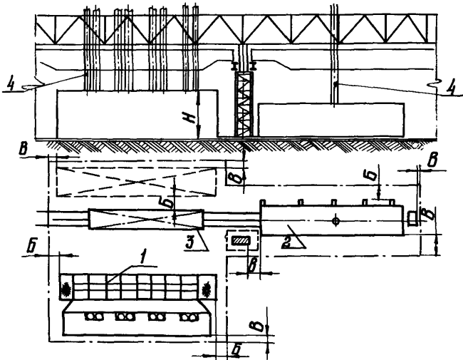
Рис.54. Размещение участка окраски конструкций на стеллажах. 1 - установка бескамерной окраски; 2 - камера сушильная конвективная t = 100-100^{\circ}\text{C} ; 3 - тележка технологическая; 4 - труба вентиляционная
