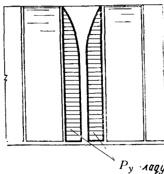
Рис. 8. Схема к расчету диафрагм массива-гиганта
