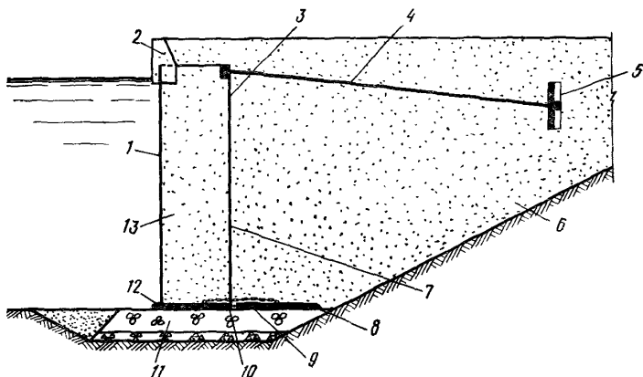
Рис. 1. Схема причального сооружения из заанкерowanych массивов-гигантов
