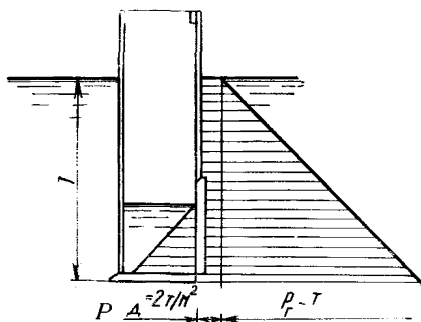
Рис. 7. Схема к расчету наружной стенки массива-гиганта
