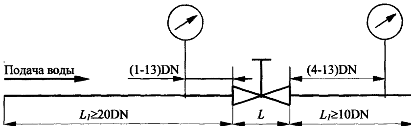
Рисунок 1 Испытательный участок стенда
