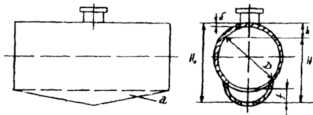
Рис. 4. Котел цистерны с выштамповкой уклона:
