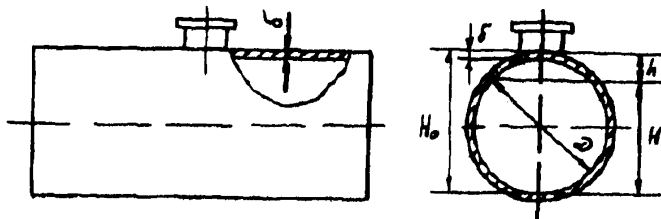
Рис. 2. Котел цистерны без ванночки и выштамповки уклона:
