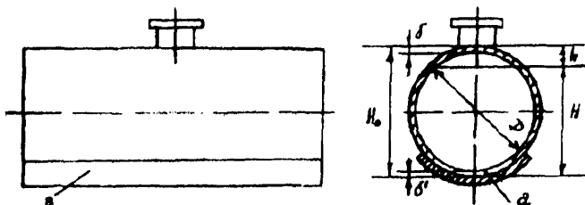
Рис. 3. Котел цистерны с ванночкой:
