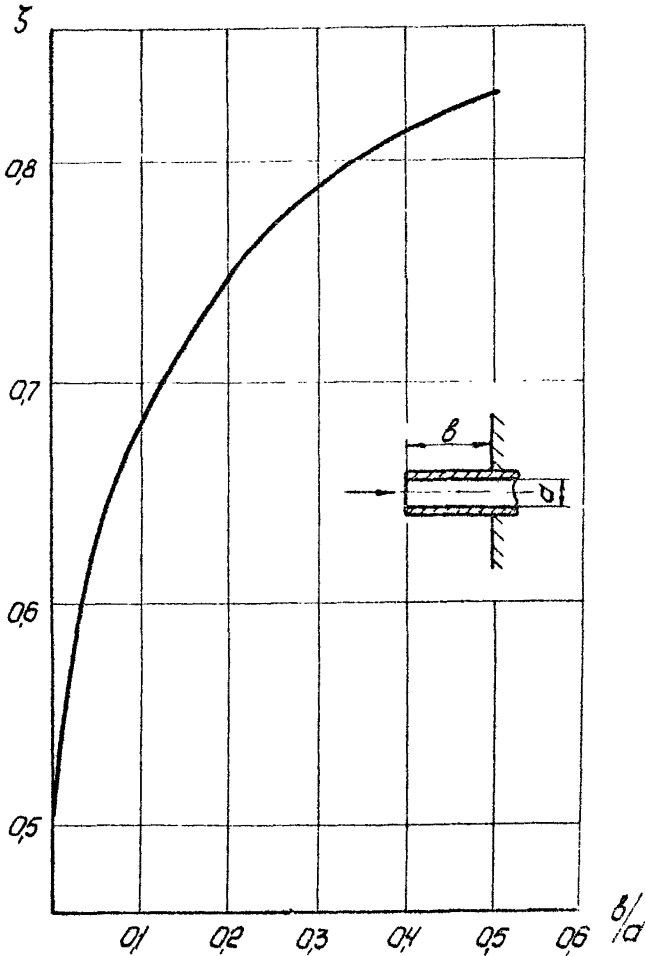
Рис. 6. Зависимость коэффициента местного сопротивления при выходе из резервуара от относительного вылета трубы ( Re = 10 \cdot 10^4 ).
