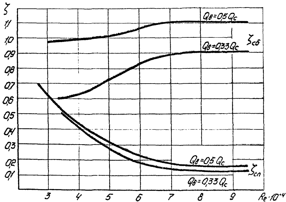
Рис. 26. Зависимость коэффициентов потерь в нагнетательном тройнике ( d_B = 7 \text{ мм} ; d_n = d_c = 100 ) от числа Рейнольдса.
