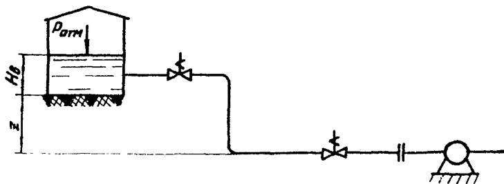
Рис.1 Расчетная схема
