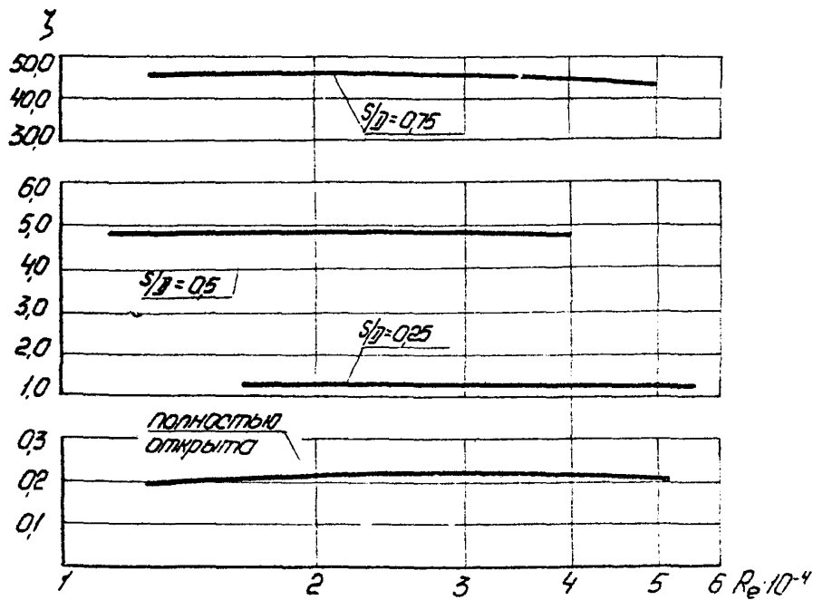
Рис. 8. Зависимость коэффициента сопротивления задвижки параллельной с разной степенью открытия S/D от числа Рейнольдса
