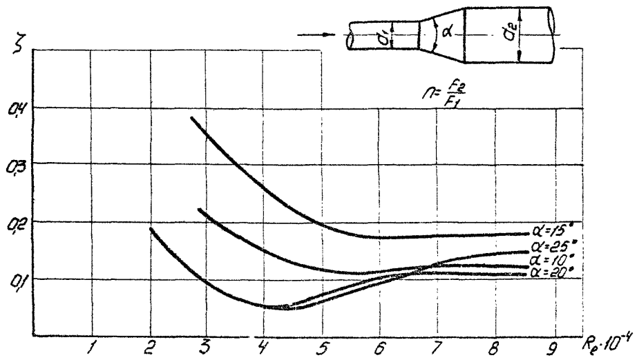
Рис. 12. Зависимость коэффициента сопротивления диффузорных переходов n = 1,96 с разными углами расширения от числа Рейнольдса.
