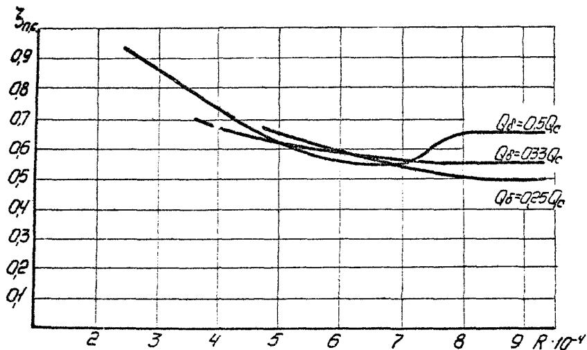
Рис. 21. Зависимость коэффициента потерь на проходе в вытяжном тройнике ( d_g = 58,5 мм; d_n = d_c = 100 мм) от числа Рейнольдса.
