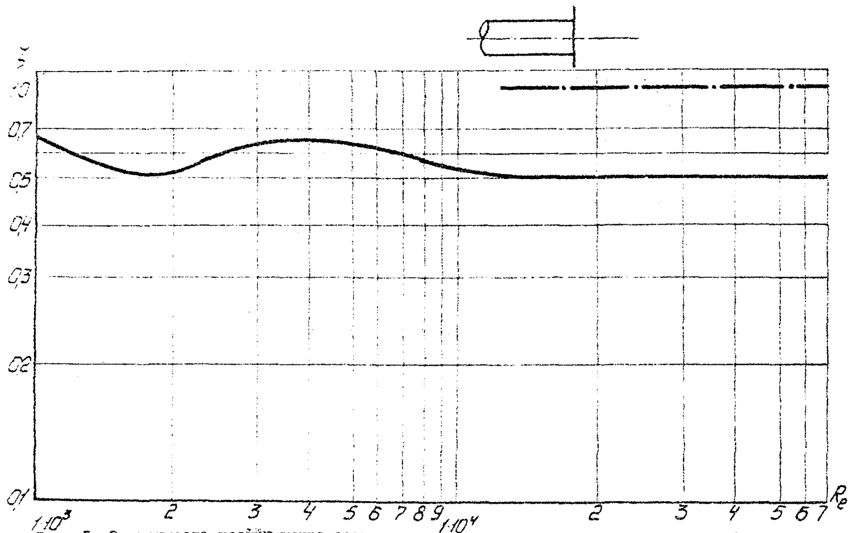
Рис. 5. Зависимость коэффициента сопротивления при выходе из резервуара в трубу, заделанную запорным вальцем в стенку; из резервуара от числа Рейнольдса ( — без хлопушки; — с хлопушкой).
