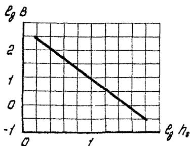
Рис. 3. Зависимость критерия тепловой кавитации от давления насыщенных паров перекачиваемой жидкости.
