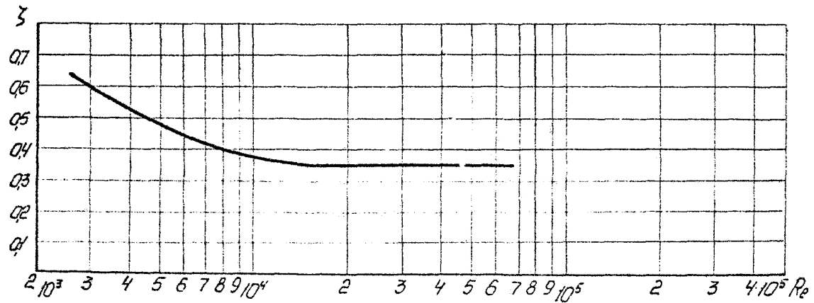
Рис. 9. Зависимость коэффициента сопротивления отвода R/D=1,5 и \delta=90^\circ (относительная шероховатость \Delta = 0,0004 ) от числа Рейнольдса.
