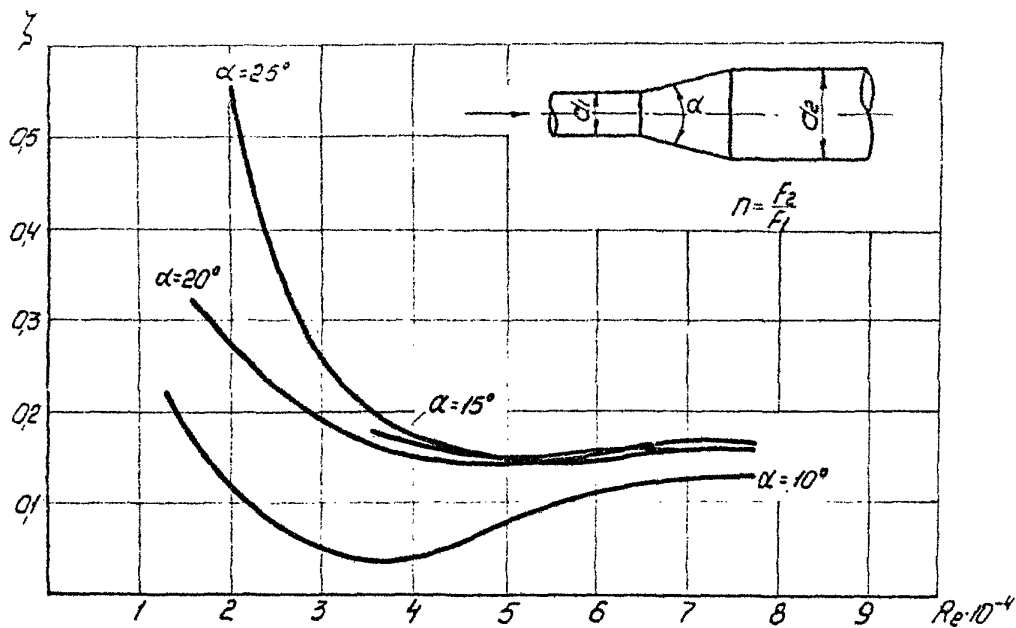
Рис. II. Зависимость коэффициента сопротивления диффузорных переходов n = 1,44 с разными углами расширения от числа Рейнольдса.
