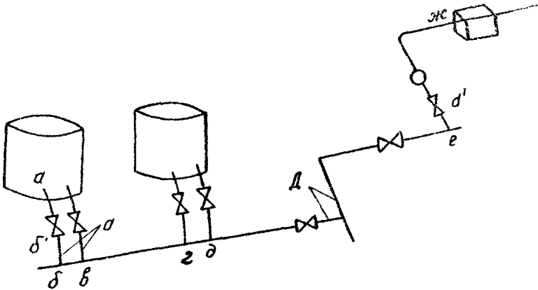
Рис 32 Расчетная схема откачки нефти из 2 х резервуаров
