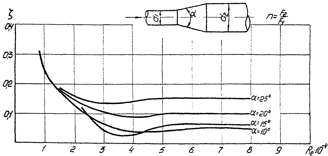
Рис. 10. Зависимость коэффициента сопротивления диффузорных переходов \eta = 1,2 с разными углами расширения от числа Рейнольдса.
