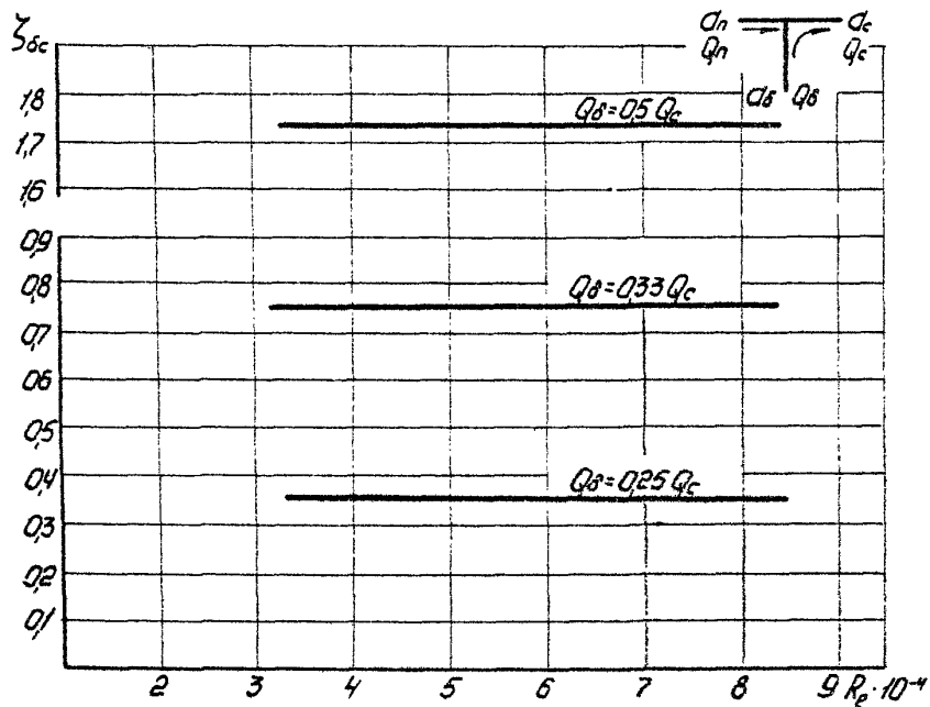
Рис. 20. Зависимость коэффициента потерь при повороте в вытяжном тройнике ( d_\delta = 58,5 мм; d_n = d_c = 100 мм) от числа Рейнольдса.
