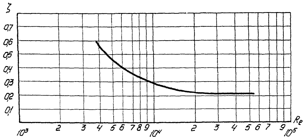
Рис. 30. Зависимость коэффициента сопротивления фильтра-решетки (степень стеснения m = 0,1 + 0,115 ) от числа Рейнольдса.
