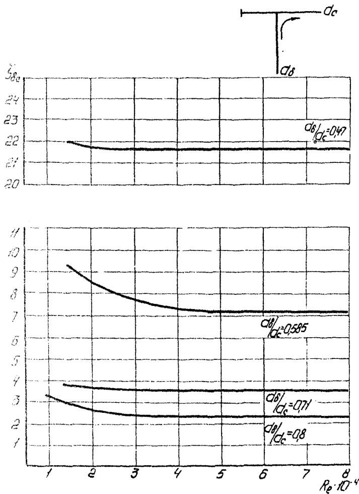
Рис. 13. Зависимость коэффициента сопротивления тройника с тупиком при повороте потока ( Q_0 = Q_c ) от числа Рейнольдса.
