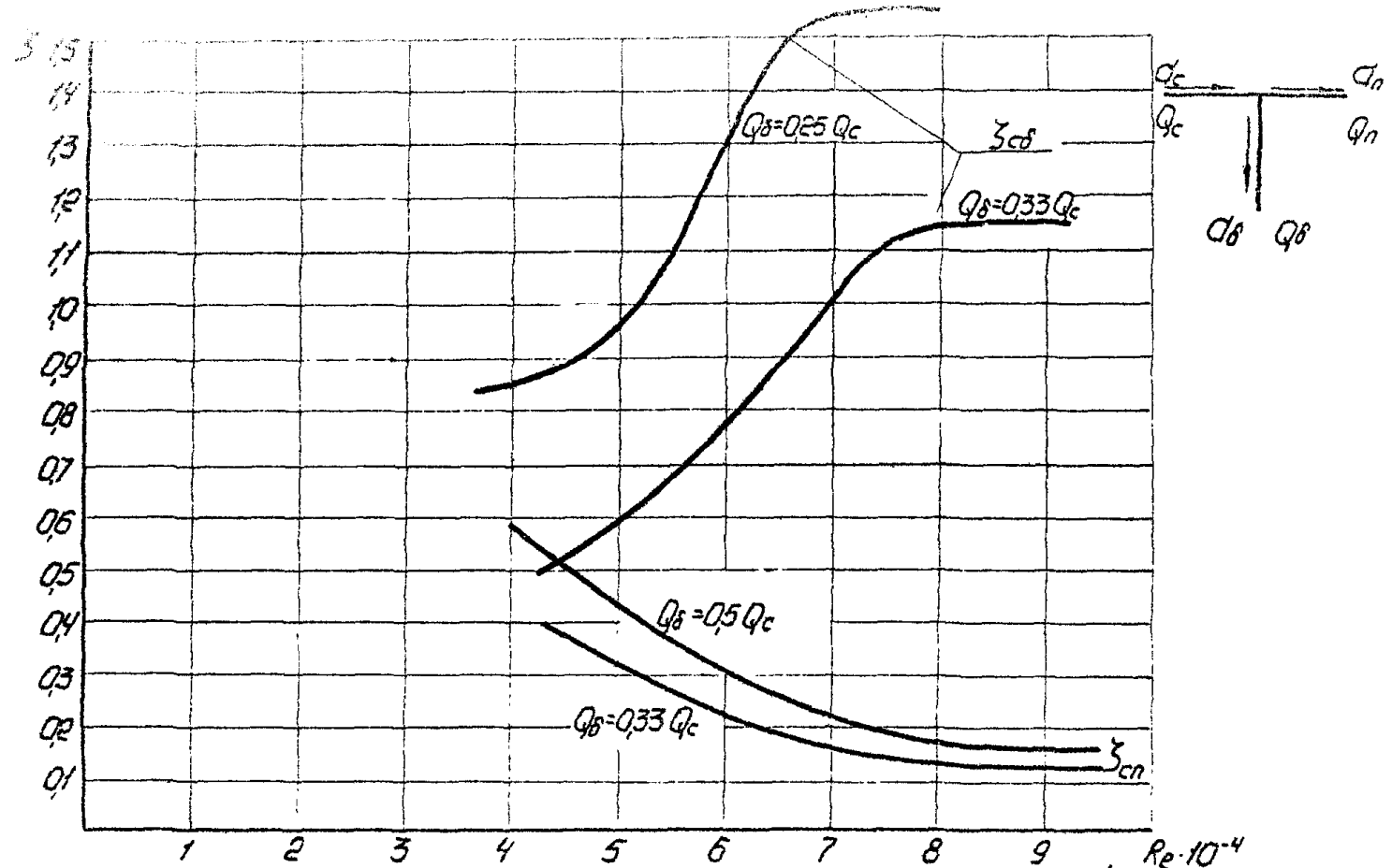
Рис. 27. Зависимость коэффициентов потерь в нагнетательном тройнике ( d_B = 58,5 мм; d_n = d_C = 100 мм) от числа Рейнольдса.
