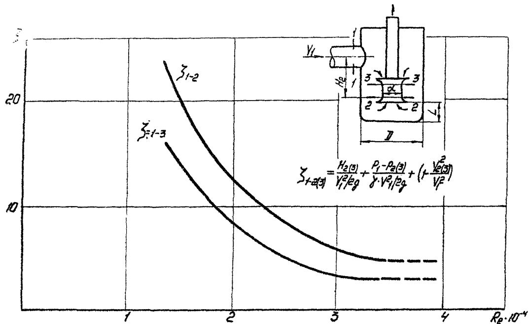
Рис. 31. Зависимость коэффициентов гидравлических потерь в стакане вертикального насоса двойного всасывания ( l/d \approx 1,0 ; d/D = 0,3 ) от числа Рейнольдса (к скорости V_1 )
