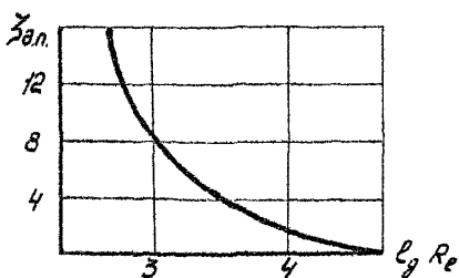
Рис. 4. Зависимость коэффициента гидравлического сопротивления от числа Рейнольдса.
