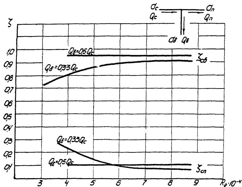
Рис. 25. Зависимость коэффициентов потерь в нагнетательном тройнике ( d_б = 80\text{мм} ; d_n = d_c = 100\text{мм} ) от числа Рейнольдса.
