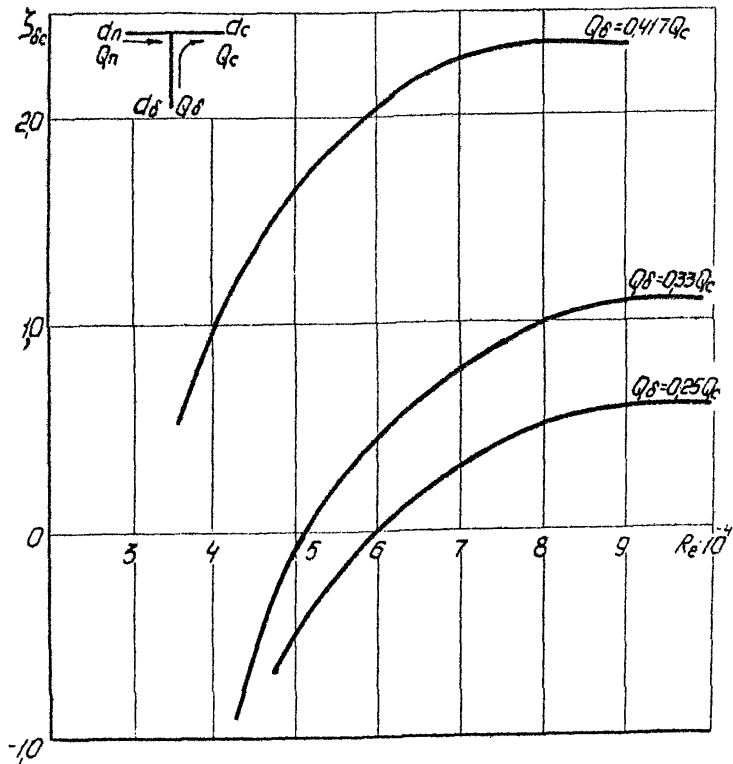
Рис. 22. Зависимость коэффициента потерь при повороте в витльном тройнике ( d_{\delta} = 47 \text{ мм} ; d_n = d_c = 100 \text{ мм} ) от числа Рейнольдса.
