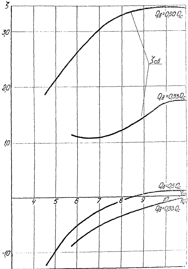
Рис. 28. Зависимость коэффициентов потерь в нагнетательной тройнике ( d_B = 47\text{мм} ; d_n = d_C = 100\text{мм} ) от числа Рейнольдса.
