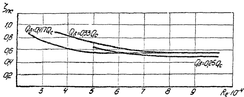
Рис. 23. Зависимость коэффициента потерь на проходе в вытяжном тройнике ( d_s = 47 мм; d_n = d_c = 100 мм) от числа Рейнольдса.
