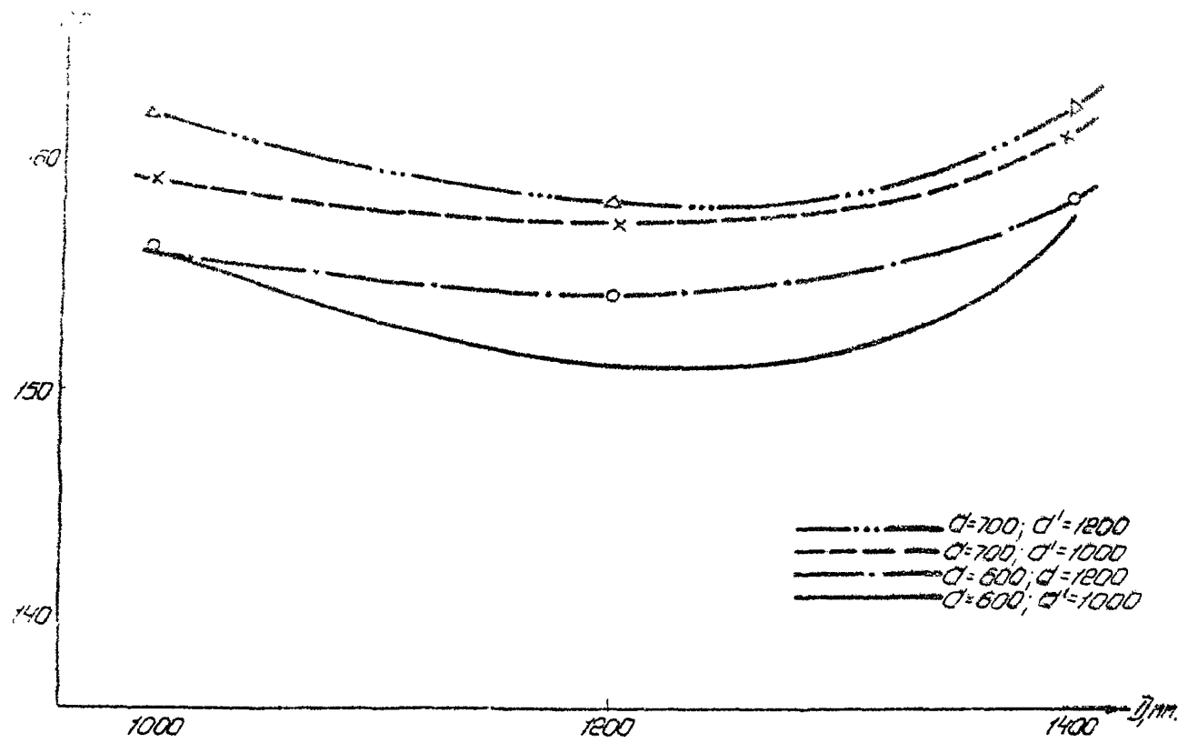
Рис. 33. Зависимость приведенных расходов от диаметров подводящих линий.
