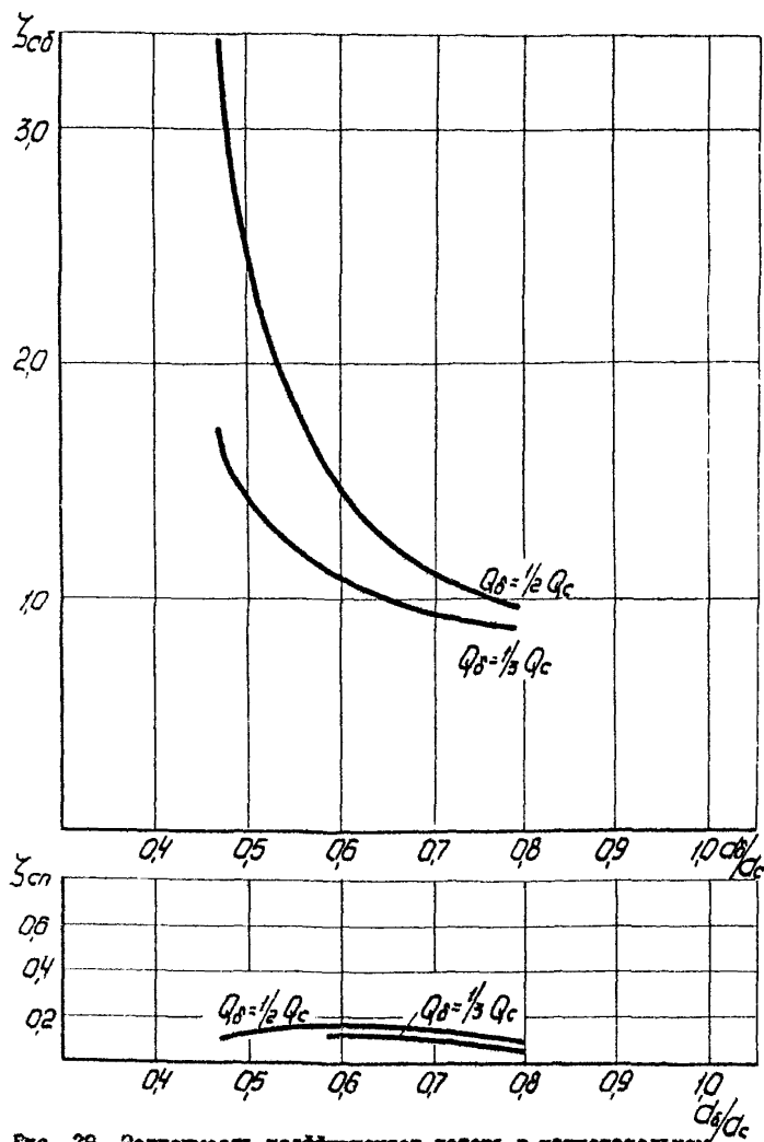
Рис. 29. Зависимость коэффициентов потерь в нагнетательном тройнике от соотношения диаметров.
