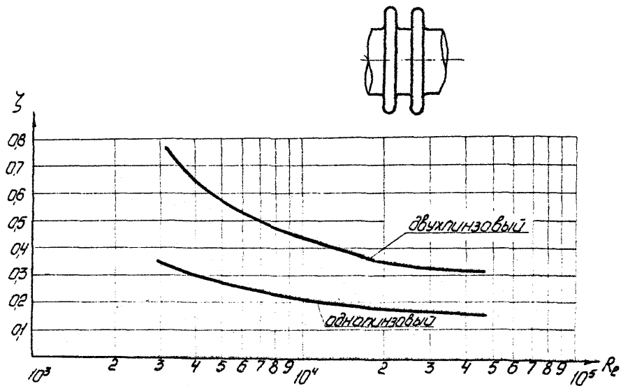
Рис. 7. Зависимость коэффициента сопротивления линзового компенсатора от числа Рейнольдса.
