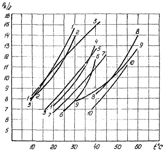
Рис. 2. Зависимость давления насыщенных паров нефтей от температуры.
