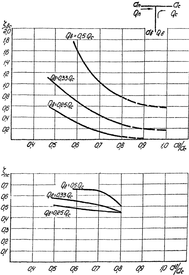
Рис. 24. Зависимость коэффициента гидравлических потерь в втяжном тройнике от отношения диаметров трубопроводов ( Re \geq 7 \cdot 9 \cdot 10^4 )
