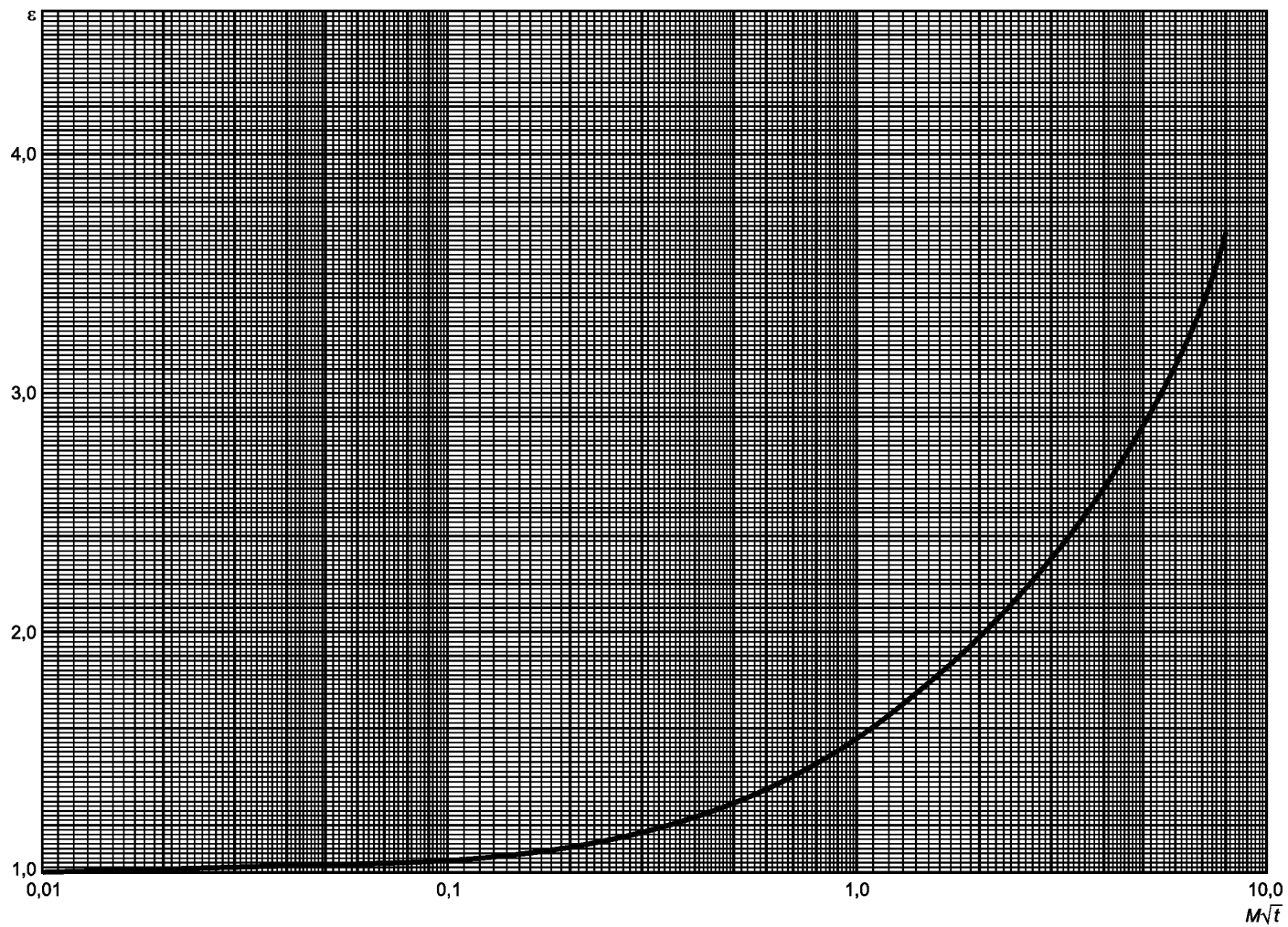
Рисунок 1 — Коэффициент \varepsilon для оболочек, экранов и брони при неадиабатическом характере нагрева
