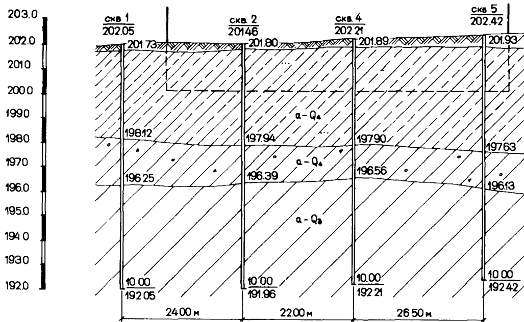
Рис.6.6. Геологический разрез 3-3
