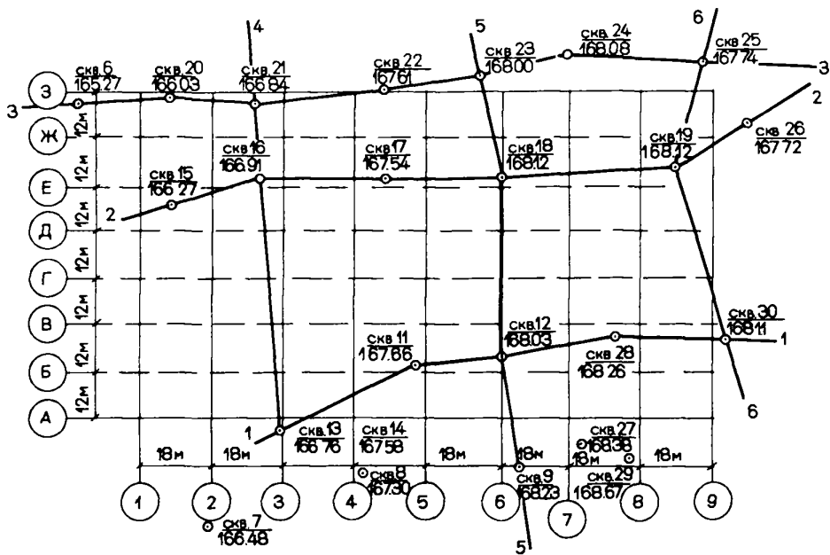
Рис.6.1. Схематический план здания и план расположения скважин
