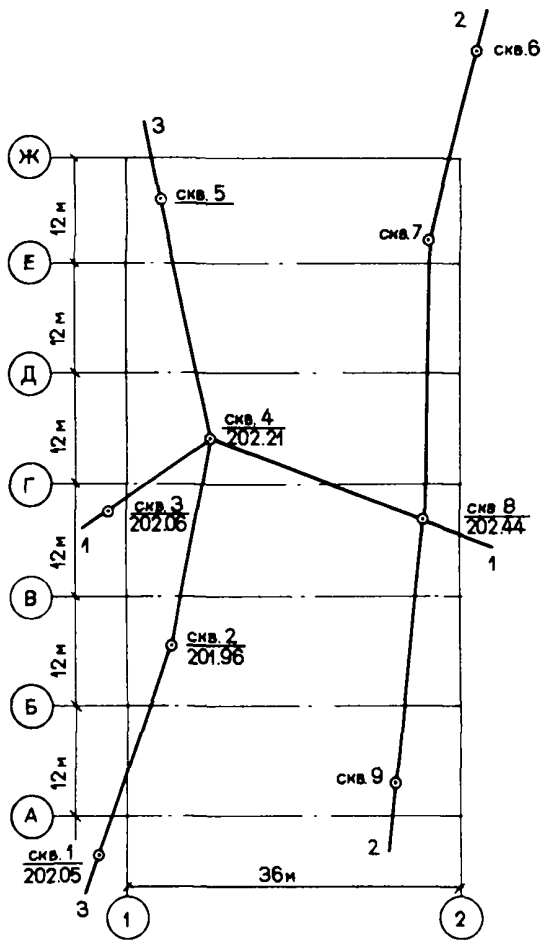
Рис.6.3. Схематический план здания и план расположения скважин
