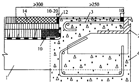
Рис. 7. Пример деформационного шва со схемой примыкания №1 и переходным участком в уровне верхнего слоя покрытия: 1 – несущая конструкция; 2 – окаймление деформационного шва; 3 – анкеровка окаймления; 4 – участок омоноличивания окаймления; 10 – дренажный канал; 12 – мастичное заполнение; 14 – переходной участок
