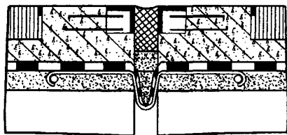
Рис. 3. Недопустимое разделение бетона амоноличивания слоем гидроизоляции
