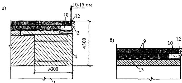
Рис. 9. Сопряжение одежды с вертикальным ребром окаймления: а – при железобетонной плите проезжей части; б – при ортотропной плите;
