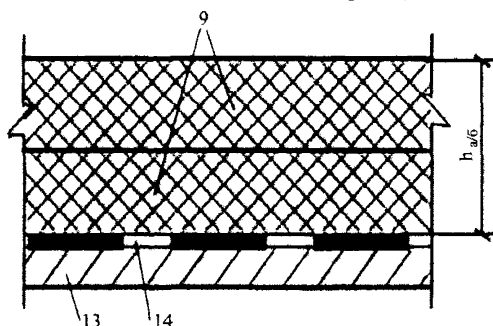
Рис. 5 Конструкция дорожной одежды на ортотропной плите: 9 – покрытие; 13 – лист ортотропной плиты; 14 – защитно-сцепляющий слой
