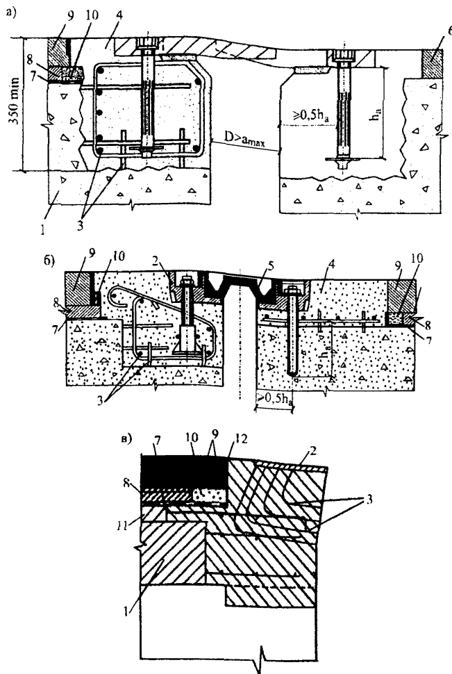
Рис. 2. Возможные схемы армирования бетонного прилива в местах анкеровки конструкций деформационных швов: 1 – несущая способность; 2 – окаймление деформационного шва; 3 – анкерка окаймления; 4 – участок амоноличивания окаймления; 5 – резиновый компенсатор; 6 – одежда ездового полотна мостового сооружения; 7 – гидроизоляция; 8 – защитный бетонный слой; 9 – покрытие; 10 – дренажный канал; 11 – выравнивающий слой; 12 – мастичное заполнение
