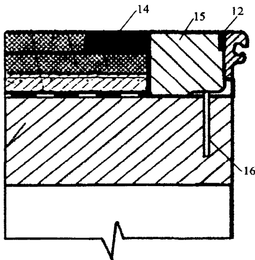
Рис. 8. Сопряжение для случая крепления окаймления «химическими анкерами»:
