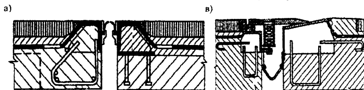
Рис. 1. Примеры заведения гидроизоляции «под козырек» окаймления
