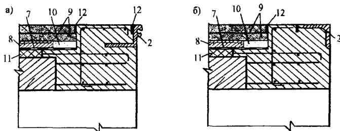
Рис. 6: 2 – окаймление деформационного шва; 7 – гидроизоляция; 8 – защитный бетонный слой; 9 – покрытие; 10 – дренажный канал; 11 – выравнивающий слой; 12 – мастичное заполнение
