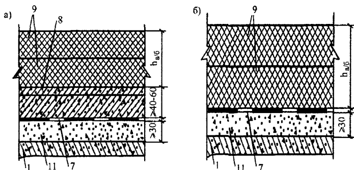
Рис. 4. Конструкция дорожной одежды:
