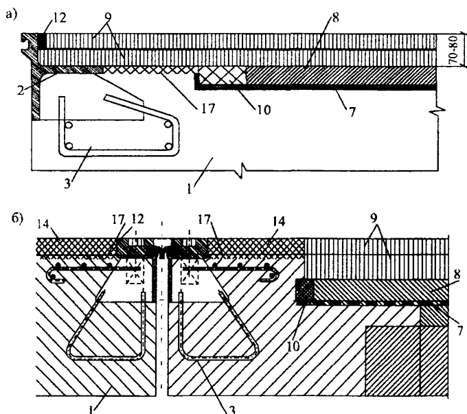
Рис. 10. Варианты примыкания дорожной одежды к деформационному шву по схеме № 4:
