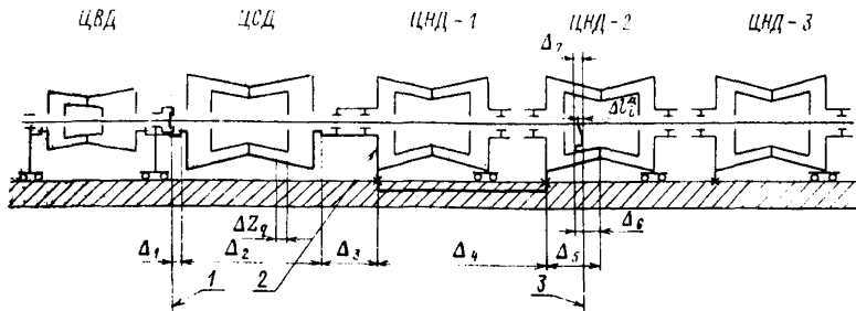
1 — плоскость прилегания рабочих колодок упорного подшипника; 2 — линия жесткой связи; 3 — расчетное сечение
