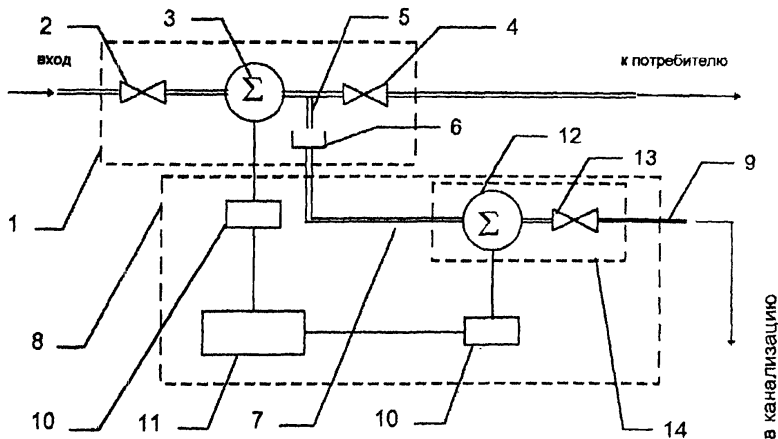
Принципиальная гидросистема узла установки счетчика воды для подключения поверочной установки "ПРОЛИВ-М"
