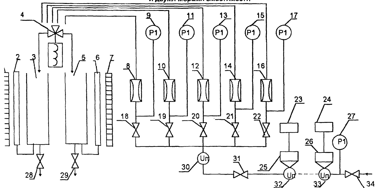
Принципиальная схема измерительной установки с оптоэлектронными узлами съема сигналов и двумя мерами вместимости
