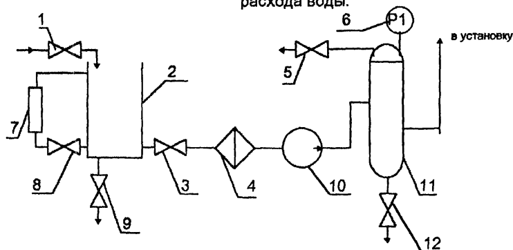
Принципиальная схема системы заправки, хранения и стабилизации расхода воды.
