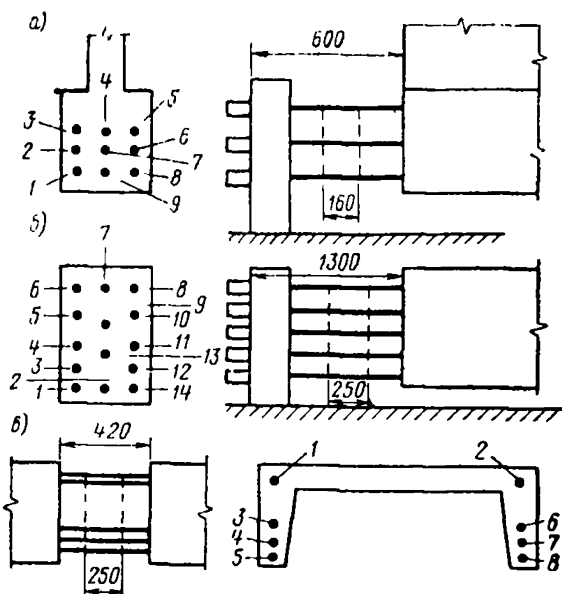
Рис. 68. Схемы разогрева свободных участков прядей с помощью газокислородного пламени
