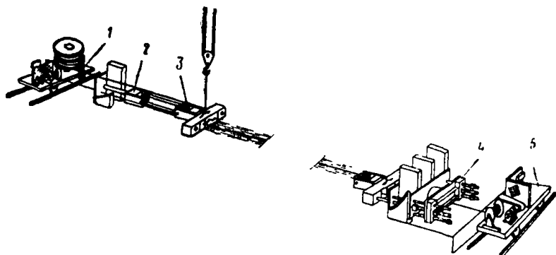
Рис. 35. Механизированная линия непрерывной раскладки и группового натяжения прядевой арматуры 1 — тележка с буктодержателями; 2 — неподвижная часть полиспаста; 3 — перемещаемая часть полиспаста; 4 — упорное и натяжное устройство стенда; 5 — тележка с лебедкой для протяжки пакета прядей
