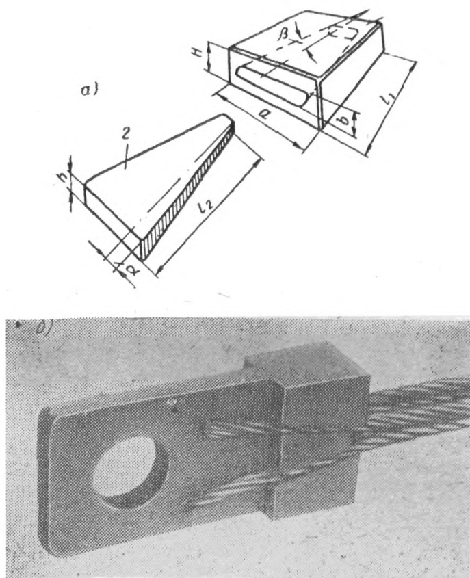
Рис. 41. Клиновые зажимы
