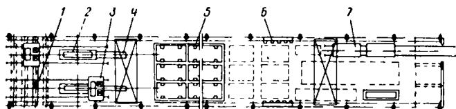
Рис. 31. Технологическая линия изготовления преднапряженных плит перекрытий размером до 3 \times 6 м
