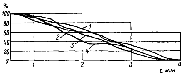
Рис. 67. Осциллограммы напряжений пакета прядей при их отпуске (одновременный нагрев прядей бензорезом)
