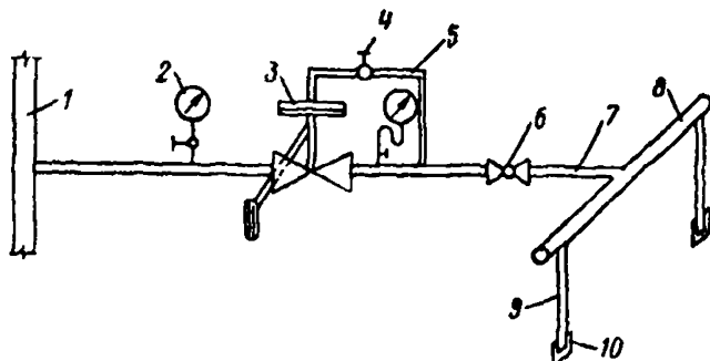
Рис. 57. Схема подачи пара в смеситель (С-336) 1 — паропровод подключения; 2 — манометр; 3 — регулятор движения; 4 — вентиль; 5 — импульсная трубка; 6 — клапан-задвижка; 7 — магистраль Ø 4'' (дюйма); 8 — коллектор Ø 4'' (дюйма); 9 — па трубок Ø 3'' (дюйма); 10 — насадка с соплами
