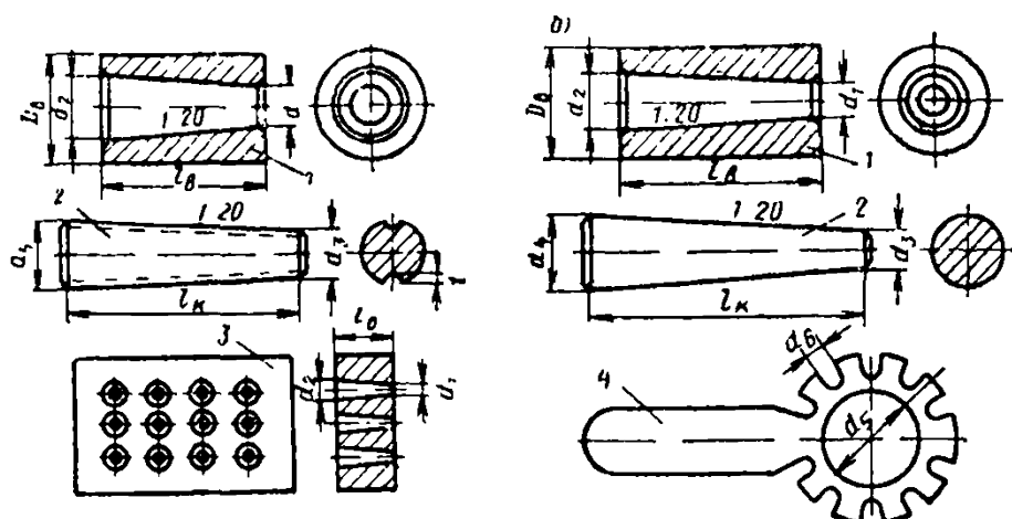
Рис. 40. Зажимы с клином для двухпрядевых канатов a — заводского изготовления; b — местного изготовления; D_{\text{в}} — наружный диаметр втулки; d_1 и d_2 — внутренние диаметры во втулке или в анкерной плите под клин; d_3 и d_4 — диаметры клина; l_{\text{к}} — длина клина; l_{\text{в}} — длина втулки или толщина анкерной плиты; t — глубина канавки; 1 — втулка; 2 — клин; 3 — анкерная плита; 4 — кондуктор (количество пазов принимается по числу проволок в канате)
