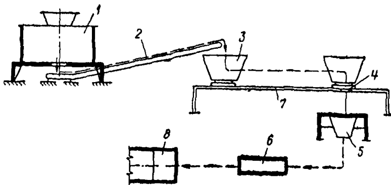
Рис. 56. Схема движения горячей бетонной смеси 1 — бетономеситель; 2 — транспортер, 3 — промежуточный бункер; 4 — перегрузка в бетоноукладчик; 5 — бетоноукладчик; 6 — формовочный пост; 7 — эстакада; 8 — пропарочные камеры
