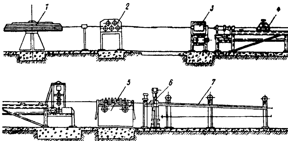
Рис. 36. Автомат для заготовки высокопрочной проволоки с высеченными концевыми и промежуточными головками (НИИЖБ)
