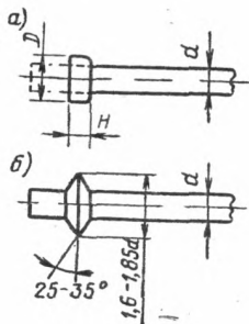
Рис. 11. Концевые (а) и промежуточные (б) высаженные головки
