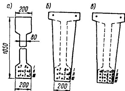
Рис. 69. Сечение преднапряженных конструкций, при изготовлении которых применялся поочередный отпуск арматуры
