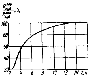
Рис. 25. Соотношение кубиковой прочности горячего и охлажденного бетона в зависимости от длительности тепловлажностной обработки
