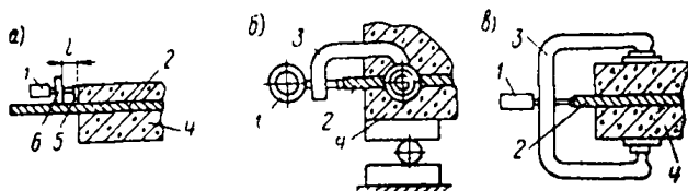
Рис. 70. Схемы крепления индикаторов для определения величины втягивания прядей в бетон
