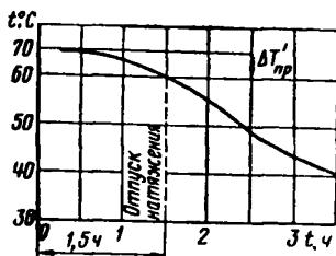
Рис. 26. Ориентировочный график остывания ферм и балок после окончания тепловлажностной обработки (температура наружного воздуха +15^{\circ}\text{C} )
