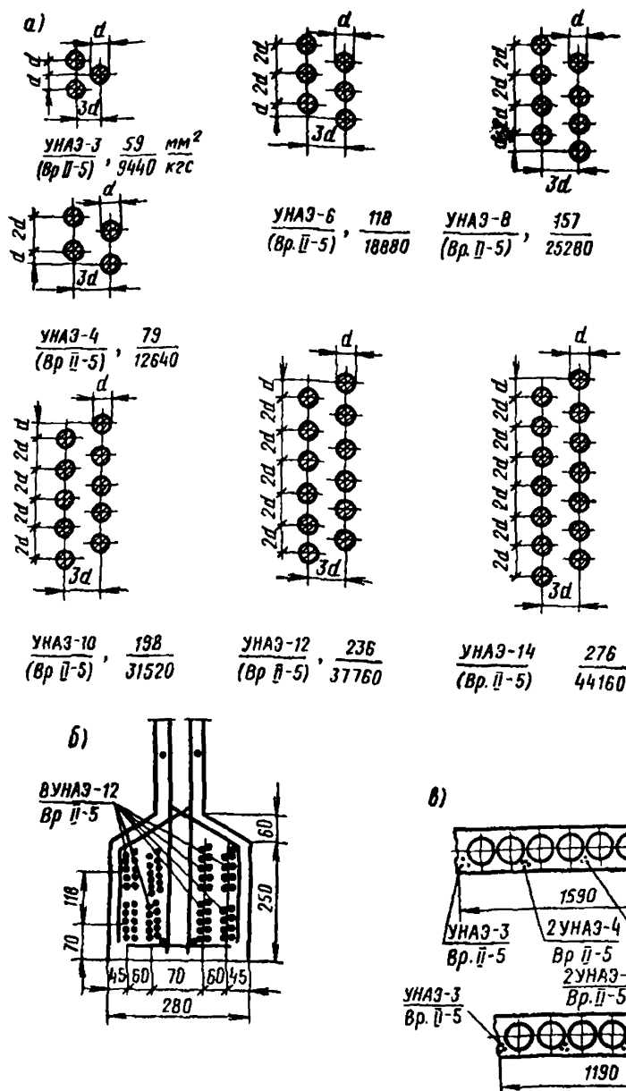
Рис. 10. Сечения и основные параметры унифицированных напрягаемых арматурных элементов (УНАЭ) и их расположение в конструкциях
