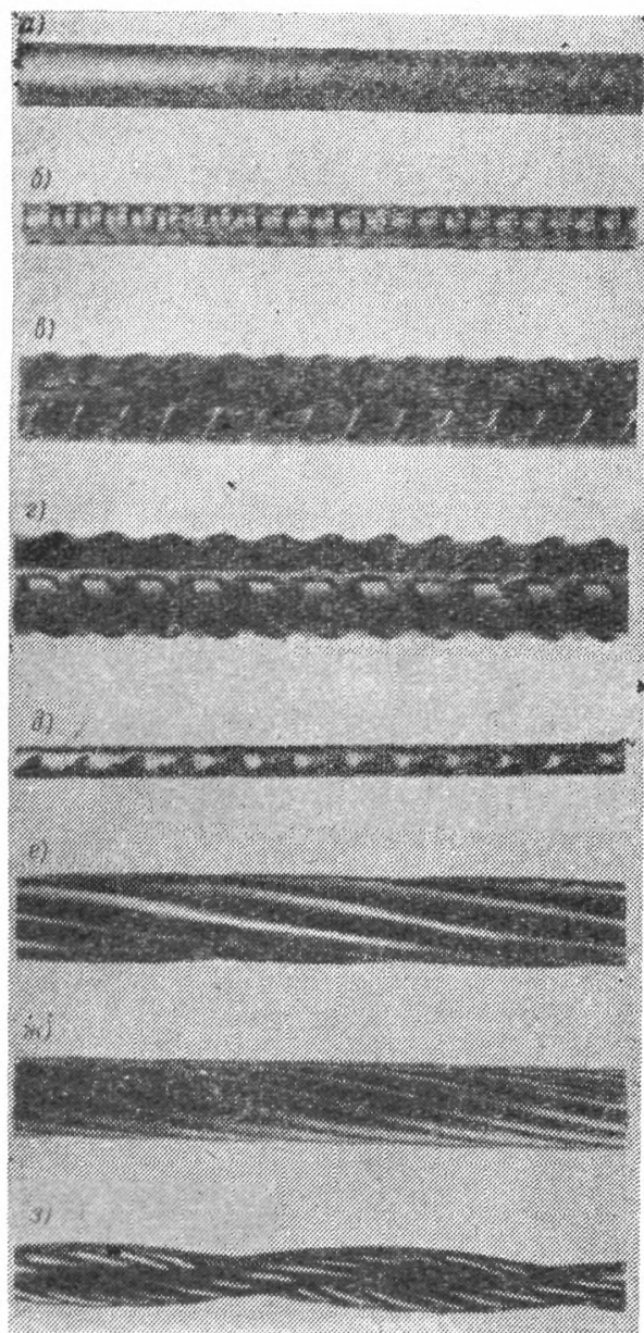
Рис. 1. Внешний вид арматурных сталей различных классов
