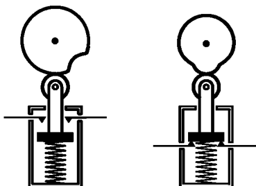
Выключатель А
