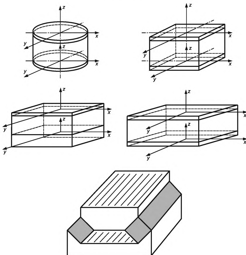
Рисунок Б.1 — Обобщенная схема осесимметричных виброизоляторов и виброизоляторов, симметричных относительно плоскостей xz и zy
