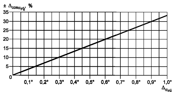
Рисунок В.1 — Зависимость максимальной погрешности \pm \Delta_{\cos \alpha_{Fq}} от угла сдвига фаз между измерительными каналами силы и скорости при \alpha_{Fq \max} = 87^\circ
