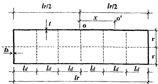
Рисунок 39 - Схема к расчету резервуара с кольцами жесткости без диафрагм
