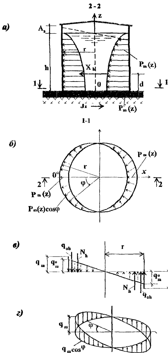
Рисунок 14 - Схема к расчету фундаментной плиты на нагрузки от гидродинамического давления
