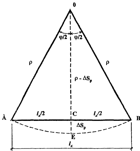
Рисунок 1 - Расчетная схема для определения дополнительных напряжений в днище от неравномерной осадки резервуара
