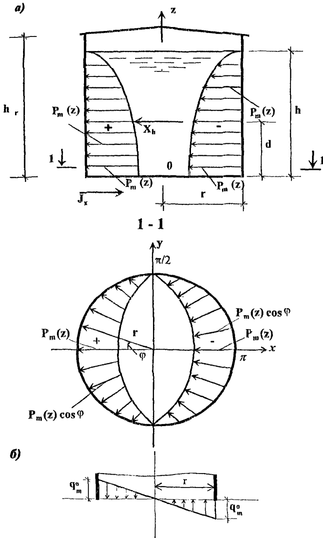
Рисунок 2 - Схема гидродинамического давления на стенку и днище резервуара при горизонтальном перемещении с ускорением от сейсмического воздействия
