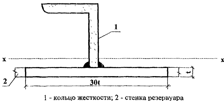
Рисунок 29 - Расчетное сечение кольца жесткости
