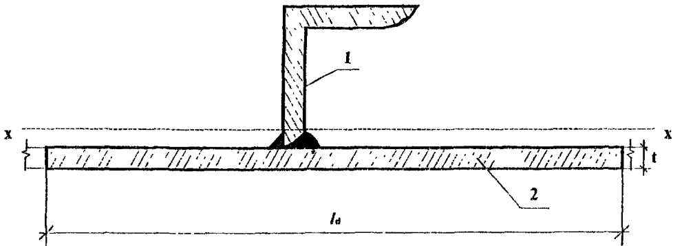
1 - кольцо жесткости; 2 - стенка резервуара
