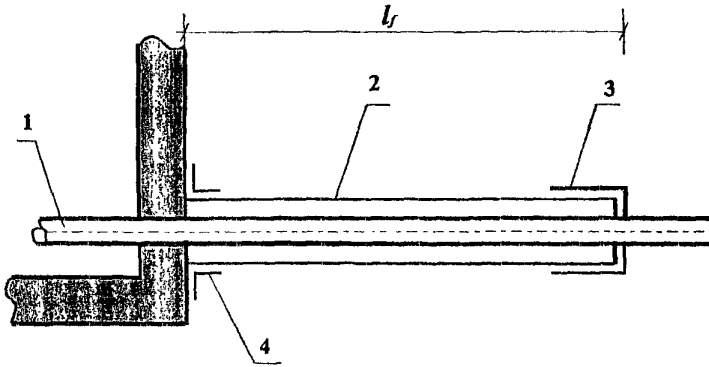
Рисунок 49 - Схема компенсационного устройства
