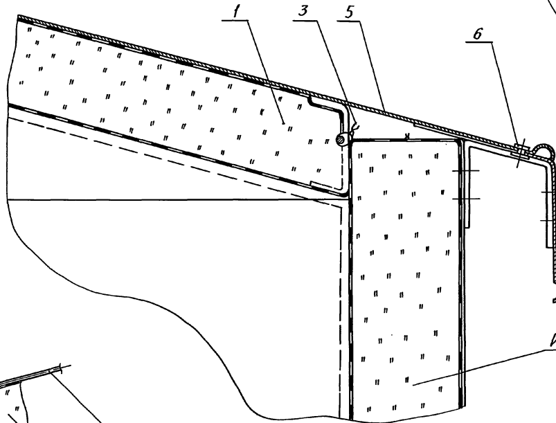
Разрез И-И лист 14
