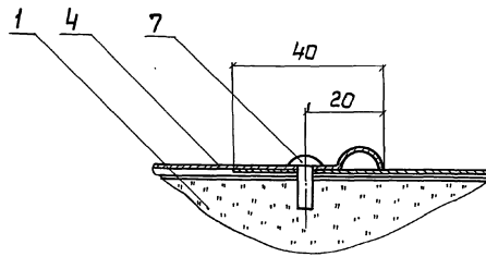
Разрез Г-Г
