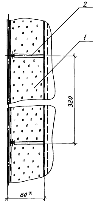
Разрез Е-Е лист 14
