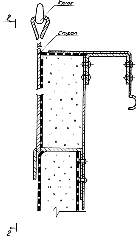
Узел строповки теплоизоляционной панели КТПП-П
