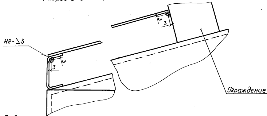
Разрез Б-Б
