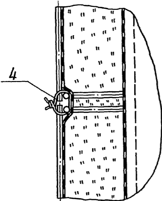
Разрез Л-Л
