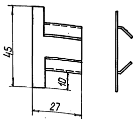
Поз.1
