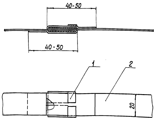
Поз.1 Развертка
