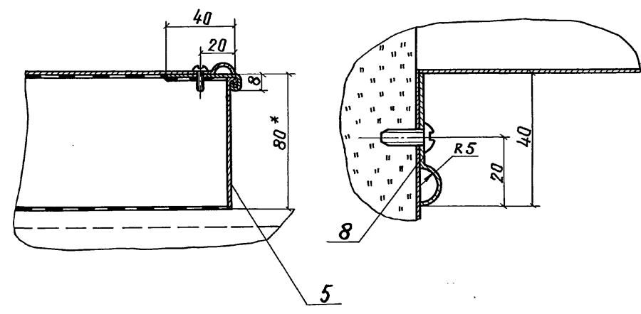
Разрез Г-Г
