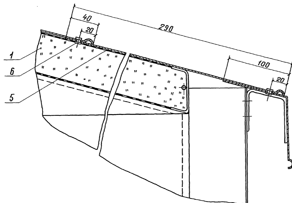
Разрез М-М повернуто
