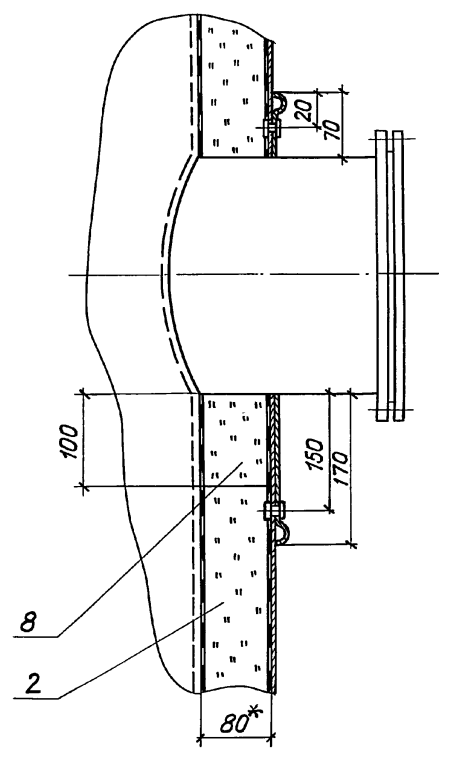
Разрез Д-Д, лист 10
