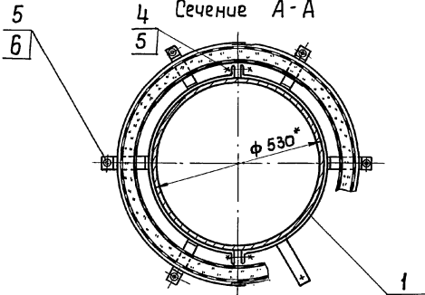
Сечение А-А
