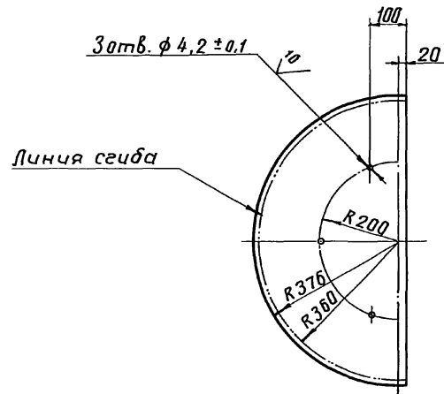
Поз. 2. Развертка
