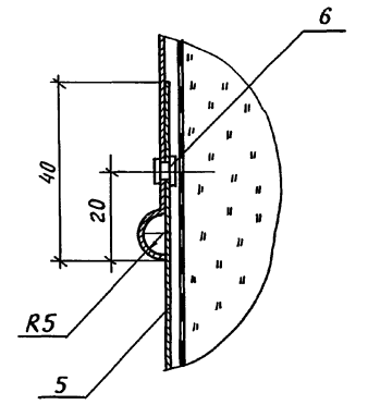
Разрез Е-Е лист 14
