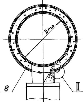
Разрез Д-Д
