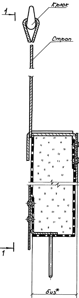
Узел строповки теплоизоляционной панели КТПП
