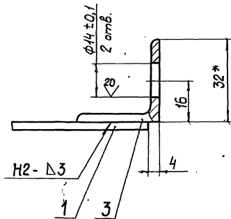
I M 1:1
