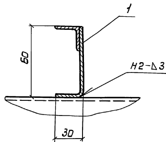
Разрез Б-Б
