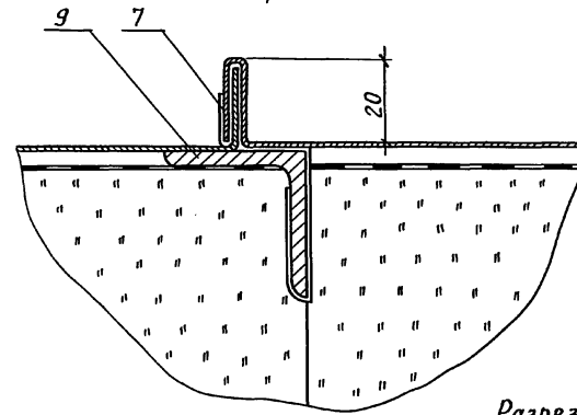
Разрез Г-Г лист
