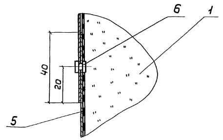
Разрез С-С
