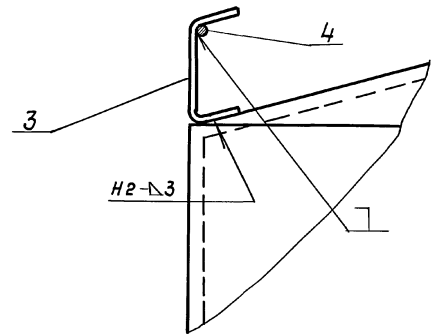
Разрез Г-Г повернуто лист 17
