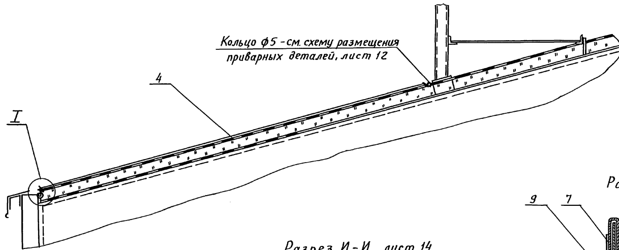
Разрез И-И лист 14
