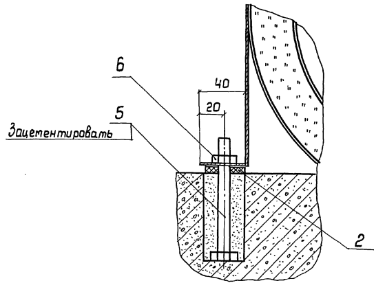
Разрез Б-Б
