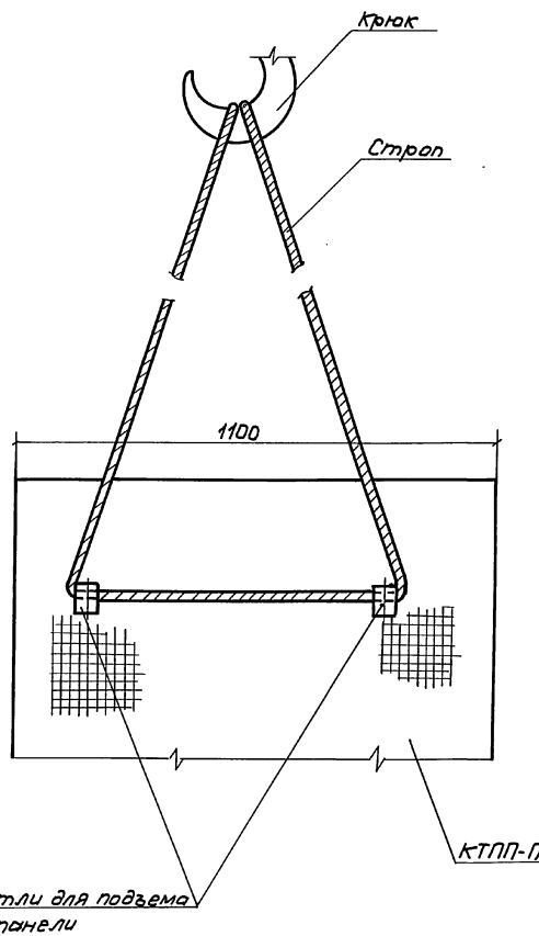
Вид 2-2
