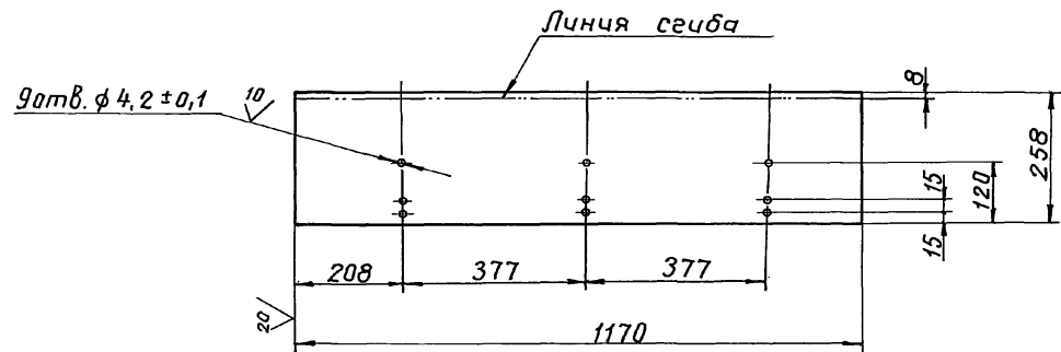
Поз. 1. Развертка
