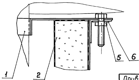
Сечение Б-Б
