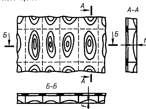
Рис. 3.4-1. Гофрировка
