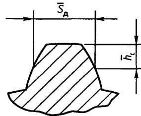
Рис. 3.2. Схема измерения толщины зуба по постоянной хорде
