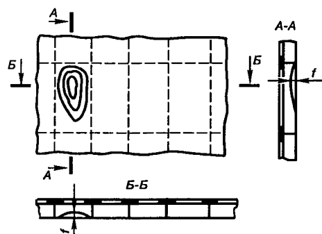
Рис. 3.4-2. Бухтина
