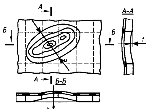
Рис. 3.4-3. Вмятина
