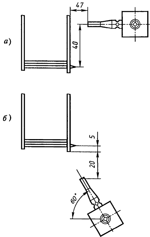
Рис. П4.2. Положение горелки относительно образца ткани
