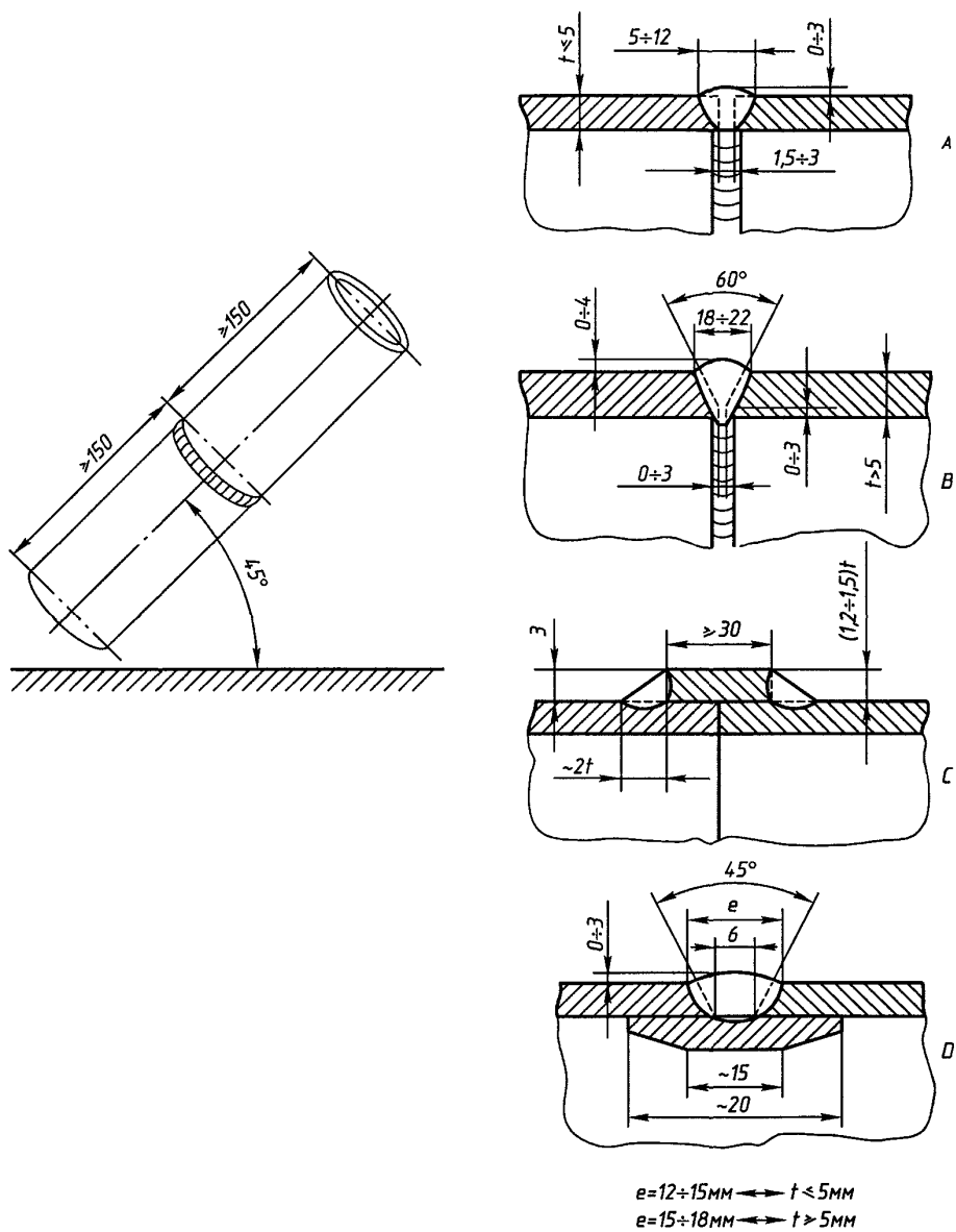
Рис. 10.2.2-6. Проба P 6
