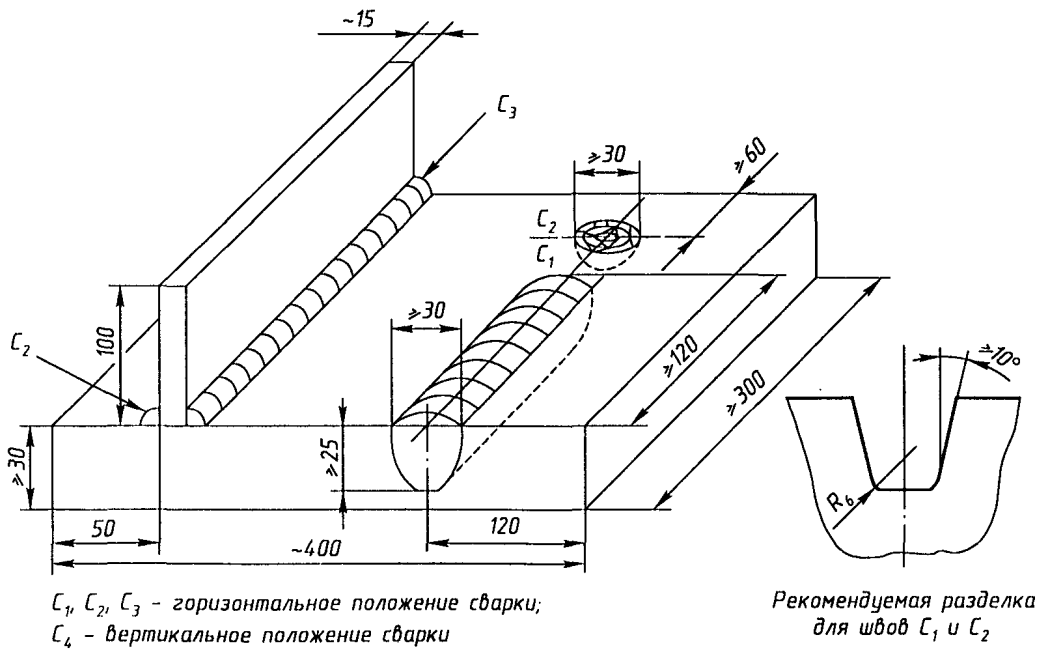
Рис. 10.2.2-8. Проба P 8
