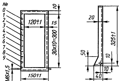
Рис. П2.2. Прибор для испытаний на распространение пламени
