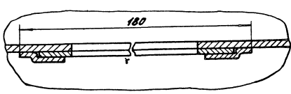
Н-Н М 1:1
