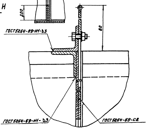
E-E М 1:1
