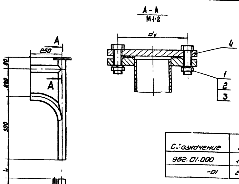
Размеры, мм
