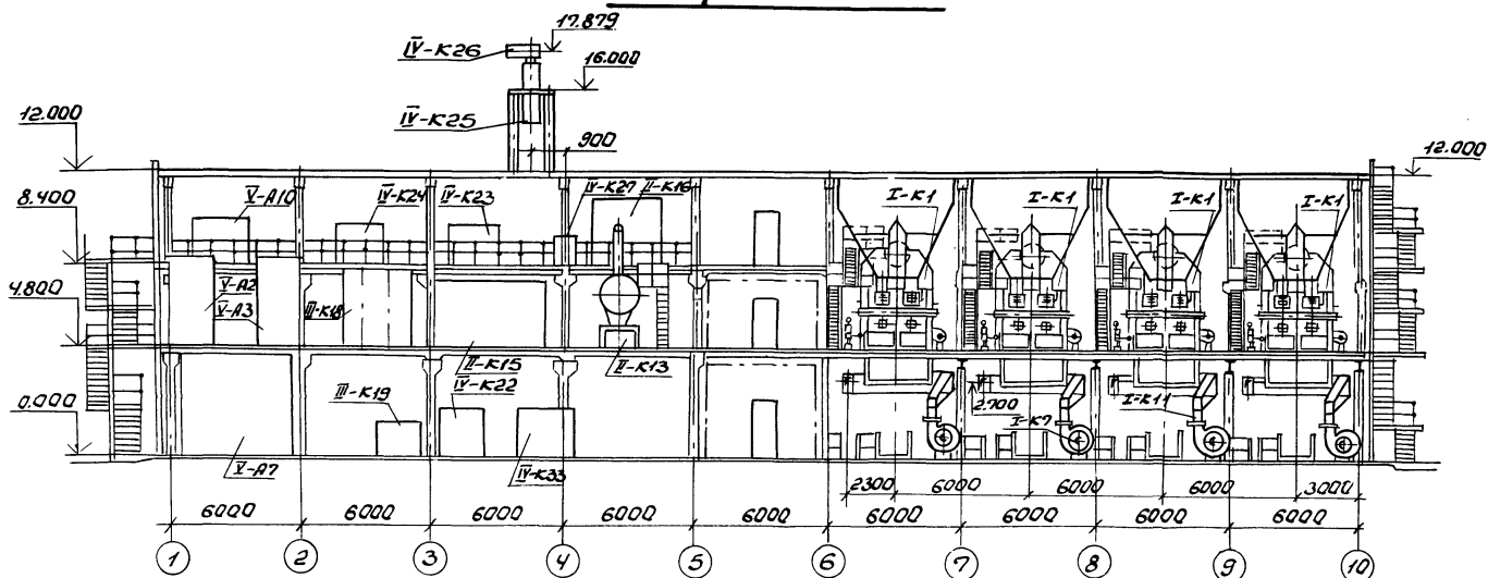
Разрез 3-3
