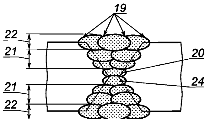
г) стыковой шов с X-образной разделкой кромок Double V-butt weld Soudure en X
