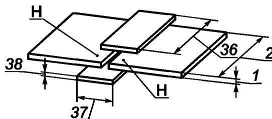
Рисунок 11 — Сборка под шовную контактную стыковую сварку по фольге
