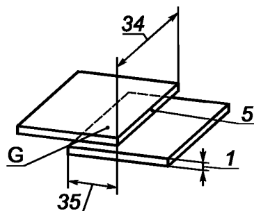
Рисунок 10 — Сборка под контактную точечную и шовную сварку с раздавливанием кромок
