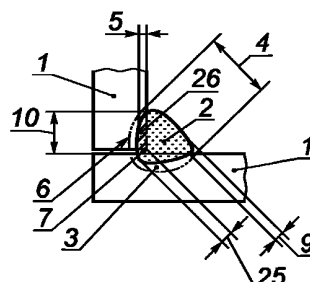
б) угловой шов Fillet weld Soudure d'angle
