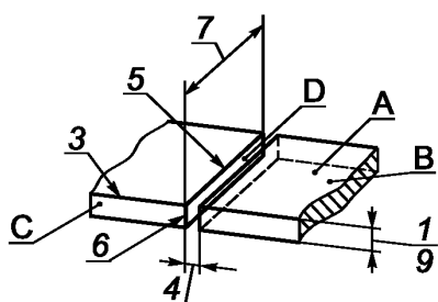
Рисунок 2 — Подготовка под сварку стыкового соединения без скоса кромок
