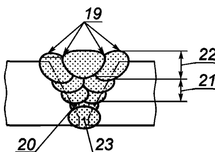
в) стыковой шов с V-образной разделкой кромок и с подварочным валиком Single V-butt weld with sealing run Soudure en V avec reprise à l'envers
