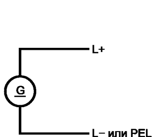
Рисунок 6 — Двухпроводная система
