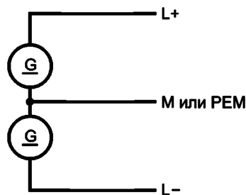
Рисунок 7 — Трехпроводная система
