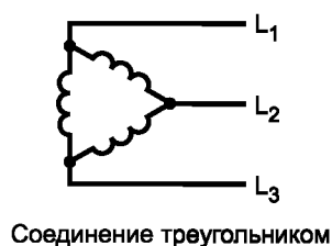
Рисунок 4 — Трехфазная трехпроводная система
