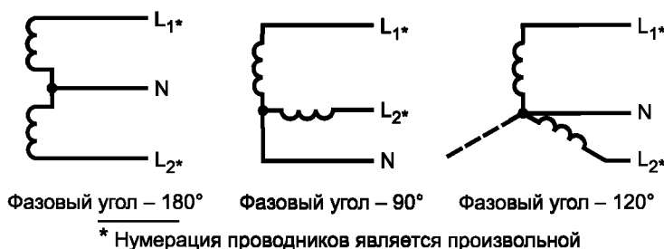
Рисунок 3 — Двухфазная трехпроводная система
