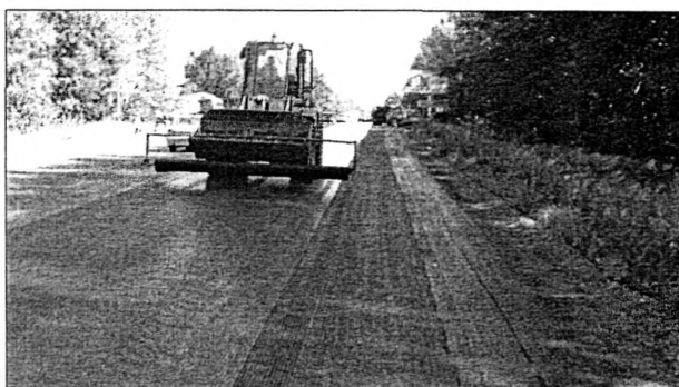
Рисунок 4. Пример укладки геосетки на основание
