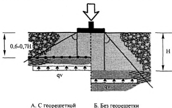
Рисунок А'. Схема, отражающая увеличение распределяющей способности щебёночного основания с георешёткой
