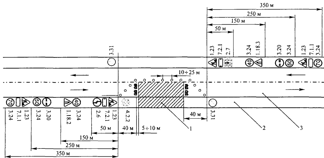
Рисунок 9. Организация ограждения места дорожных работ: 1 — зона работ; 2 — зона, примыкающая к проезжей части (обочина, газон, разделительная полоса); 3 — проезжая часть
