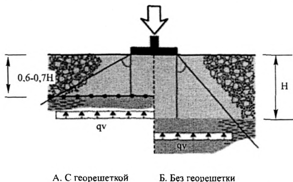
Рисунок А'. Схема, отражающая увеличение распределяющей способности щебёночного основания с георешёткой
