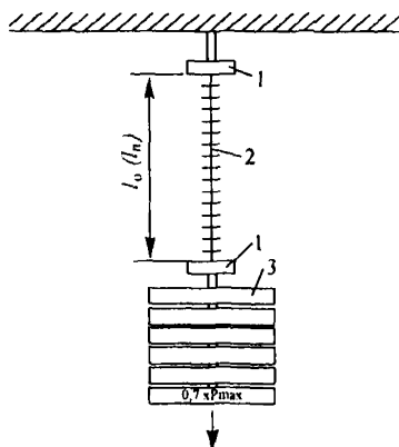
Рисунок Б у1 . Схема испытания ГМ на длительную прочность
