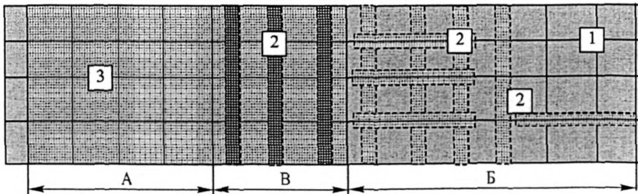
Рисунок 2. Схемы укладки геосетки (геокомпозита): A – сплошная; B – участковая; B – комбинированная; 1 – «старое» покрытие со швами (трещинами); 2 – полосы геосетки; 3 – полотно геосетки
